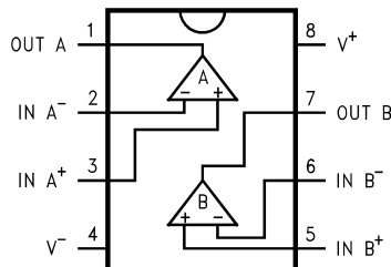
图 6-2. D 和 DGK 封装 8 引脚 SOIC、VSSOP 俯视图
