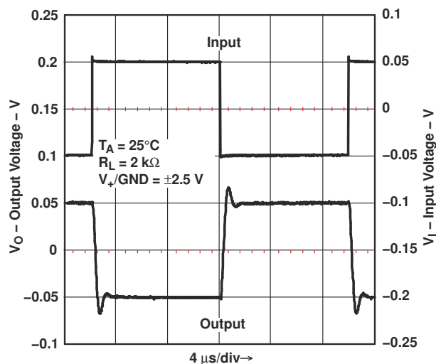
图 6-33. 小信号反相应
