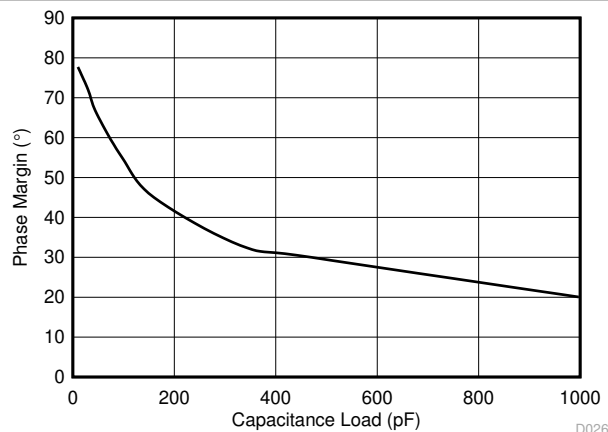
图 5-21. 相位裕度与容性负载间的关系
