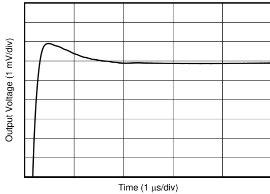
图 5-25. 大信号阶跃响应
