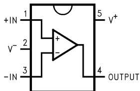
图 6-1. DBV 和 DCK 封装 5 引脚 SC70、SOT-23 俯视图
