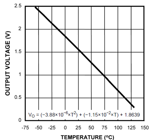
输出电压与温度间的关系
