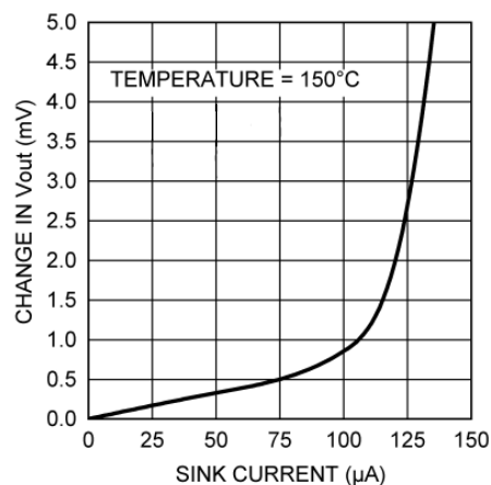
图 7-6. 负载调节，灌电流
