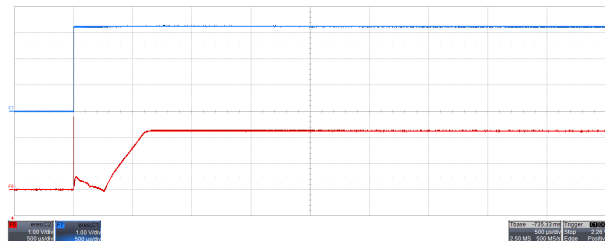
时间：500 \mu\text{s}/\text{div} ；顶部迹线： V_{DD} 1V/div；底部迹线：输出 1V/div 图 9-4. 输出导通响应时间：无容性负载， V_{DD} = 3.3\text{V}
