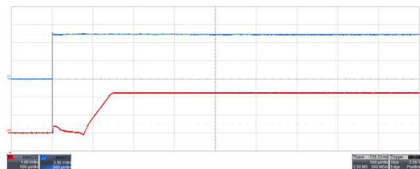
时间：500 \mu\text{s}/\text{div} ；顶部迹线： V_{DD} 2V/div；底部迹线：输出 1V/div 图 9-6. 输出导通响应时间：无容性负载， V_{DD} = 5\text{V}
