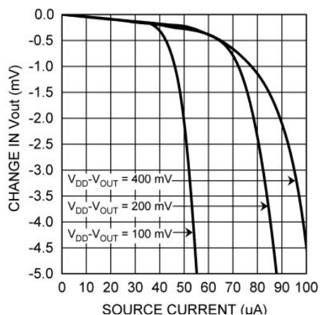
图 7-5. 负载调节，拉电流
