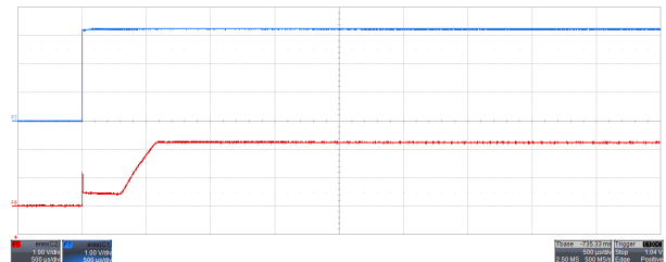
时间：500 \mu\text{s}/\text{div} ；顶部迹线： V_{DD} 1V/div；底部迹线：输出 1V/div 图 9-5. 输出导通响应时间：带 1.1nF 容性负载， V_{DD} = 3.3\text{V}
