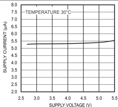
图 7-4. 电源电流与电源电压间的关系
