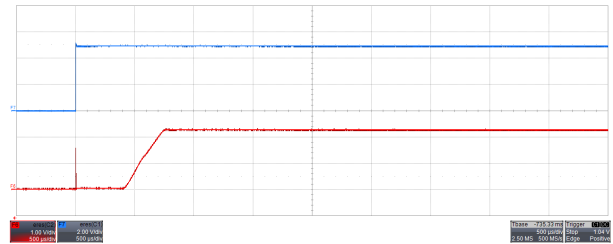
时间：500 \mu\text{s}/\text{div} ；顶部迹线： V_{DD} 2V/div；底部迹线：输出 1V/div 图 9-7. 输出导通响应时间：带 1.1nF 容性负载， V_{DD} = 5\text{V}
