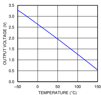
图 9-2. 模拟输出传递函数
