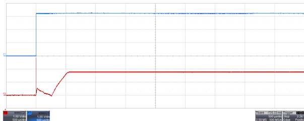
时间：500μs/div；顶部迹线： V_{\text{DD}} 1V/div；底部迹线：输出 1V/div 图 9-4. 输出导通响应时间：无容性负载， V_{\text{DD}} = 3.3\text{V}
