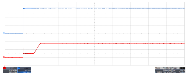
时间：500μs/div；顶部迹线： V_{\text{DD}} 1V/div；底部迹线：输出 1V/div 图 9-5. 输出导通响应时间：带 1.1nF 容性负载， V_{\text{DD}} = 3.3\text{V}
