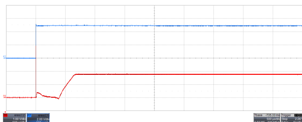
时间：500μs/div；顶部迹线： V_{\text{DD}} 2V/div；底部迹线：输出 1V/div 图 9-6. 输出导通响应时间：无容性负载， V_{\text{DD}} = 5\text{V}
