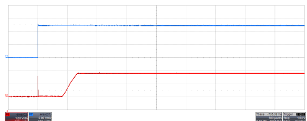
时间：500μs/div；顶部迹线： V_{\text{DD}} 2V/div；底部迹线：输出 1V/div 图 9-7. 输出导通响应时间：带 1.1nF 容性负载， V_{\text{DD}} = 5\text{V}
