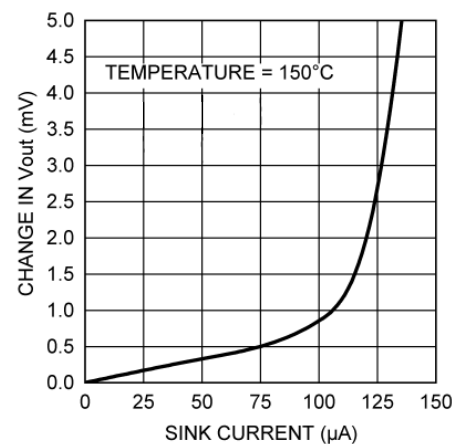
图 6-6. 负载调节, 灌电流
