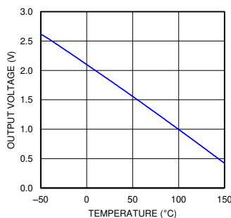
图 8-2. 模拟输出传递函数
