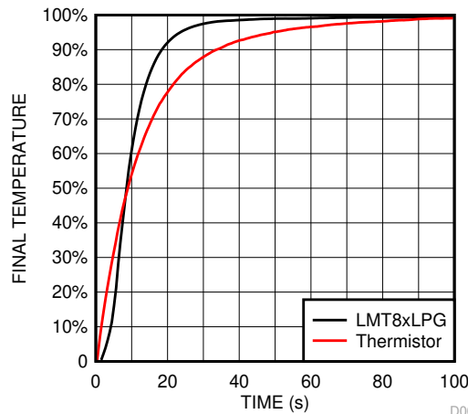
图 6-10. LMT86LPG 热响应与 1.2m/s 气流下普通引线式热敏电阻间的关系
