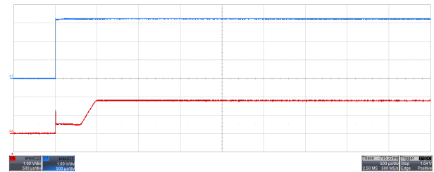
图 8-5. 输出导通响应时间：带 1.1nF 容性负载， V_{\text{DD}} = 3.3\text{V}
