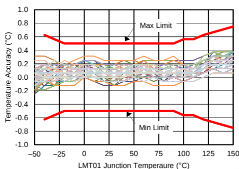
LMT01-Q1 精度
