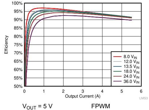
图 9-6. Efficiency
