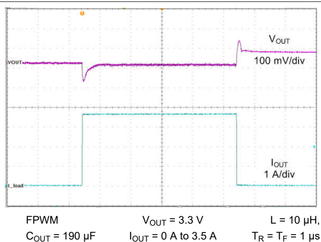
图 9-28. Load Transient
