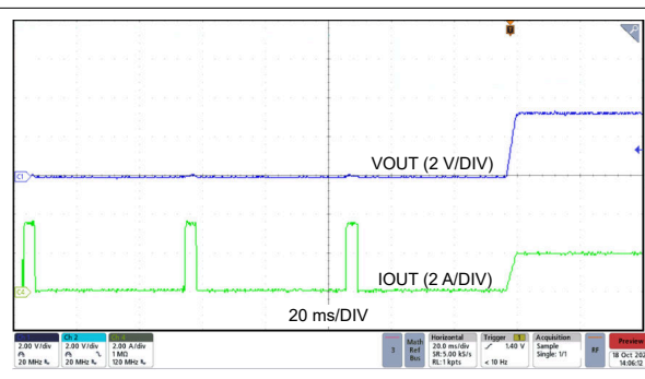
图 7-15. 退出断续
