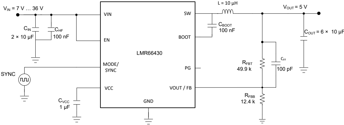
图 8-19. 应用电路 2 - 5V ( 可调 ) , 3A , 400kHz
