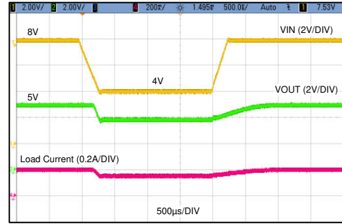
图 7-12. 典型输出从 压降中恢复 (8V 至 4V)
