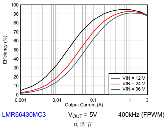
图 8-20. 效率
