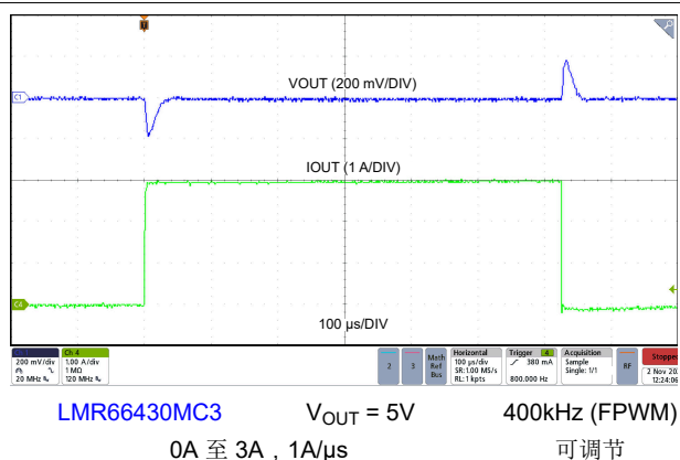
图 8-23. 负载瞬态
