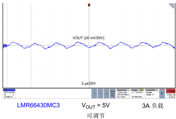
图 8-25. 输出电压纹波
