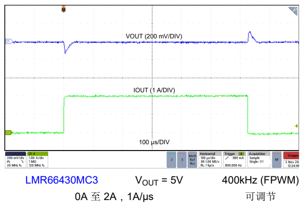
图 8-24. 负载瞬态
