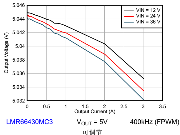
图 8-21. 线性 and 负载调整率
