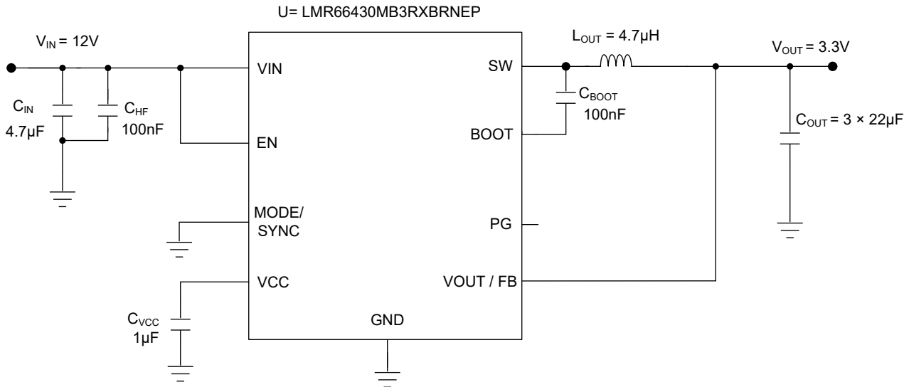
图 8-1. LMR66430-EP、1MHz (固定) 3.3V 应用电路
