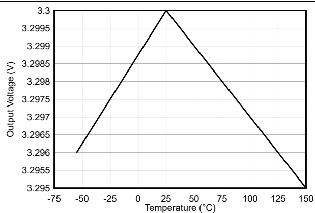
图 6-2. 输出电压精度与温度间的关系
