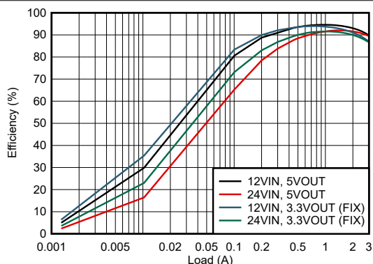
图 8-6. LMR66430MB3RBXNEP 效率 (模式 = FPWM)
