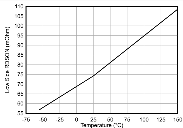
图 6-4. 低侧 MOSFET 导通电阻 ( R_{DS(on)-LS} ) 与温度间的关系
