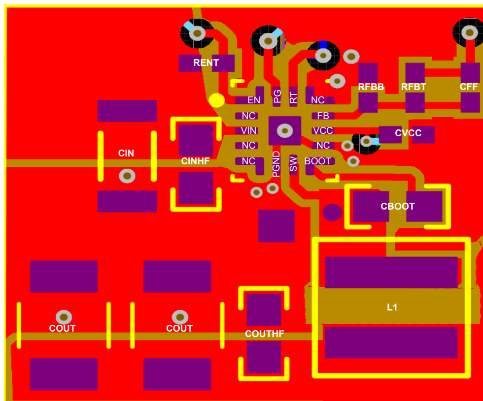
图 8-15. 示例布局
