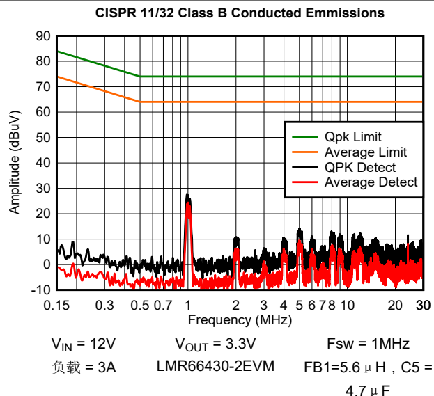
图 8-13. CISPR 11/32, B 类, 传导 EMI
