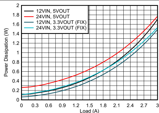
图 8-7. LMR66430MB3RBXNEP 功率耗散 (模式 = FPWM)
