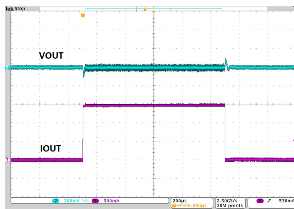
LMR66430MB3RBXNEP V_{OUT} = 3.3V (固定值) 0A 至 1.5A, 1A/μs 模式 = FPWM
