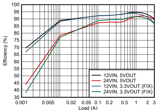
图 8-4. LMR66430MB3RBXNEP 效率 (模式 = 自动)
