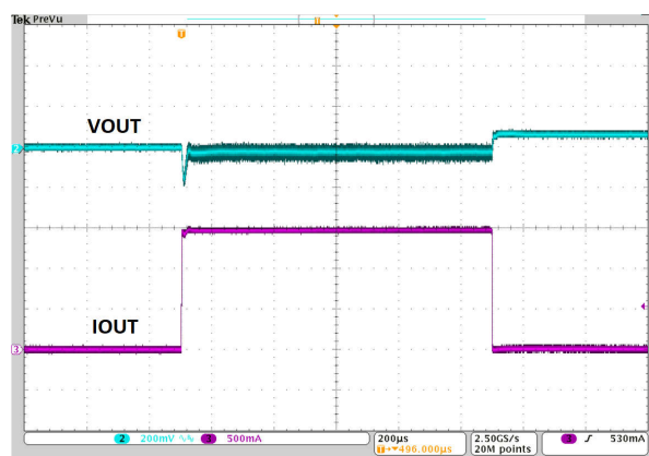
LMR66430MB3RBXNEP V_{OUT} = 3.3V (固定值) 0A 至 1.5A, 1A/μs 模式 = 自动
