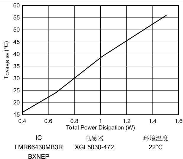
图 8-12. LMR66430-2EVM 热性能
