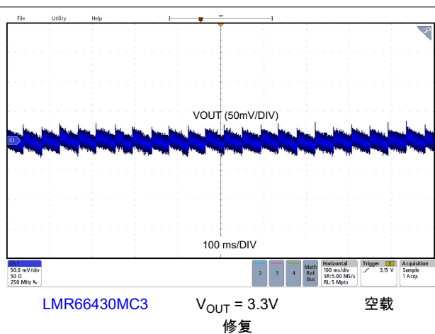
图 8-15. 输出电压纹波
