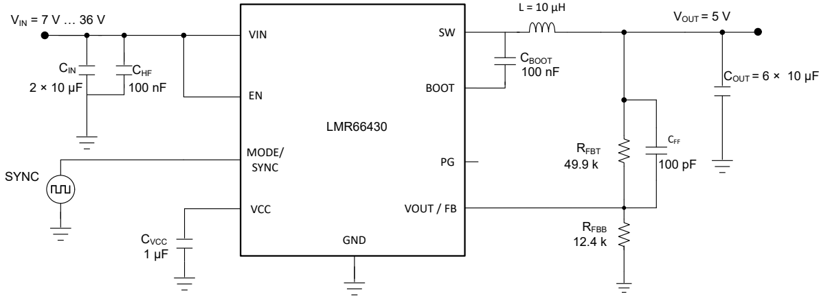
图 8-19. 应用电路 2 - 5V ( 可调 ) , 3A , 400kHz
