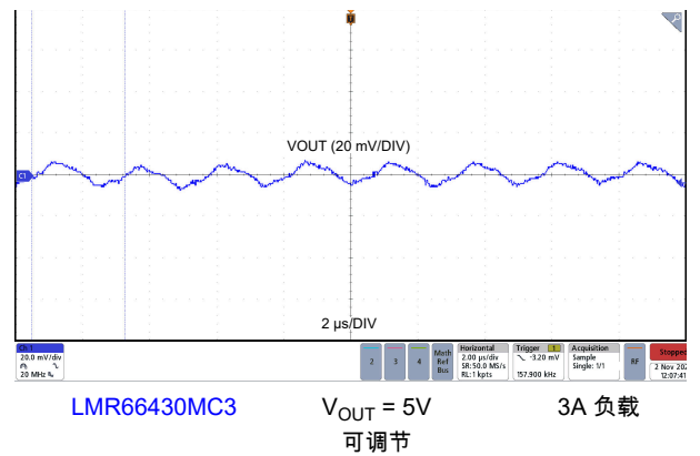
图 8-25. 输出电压纹波
