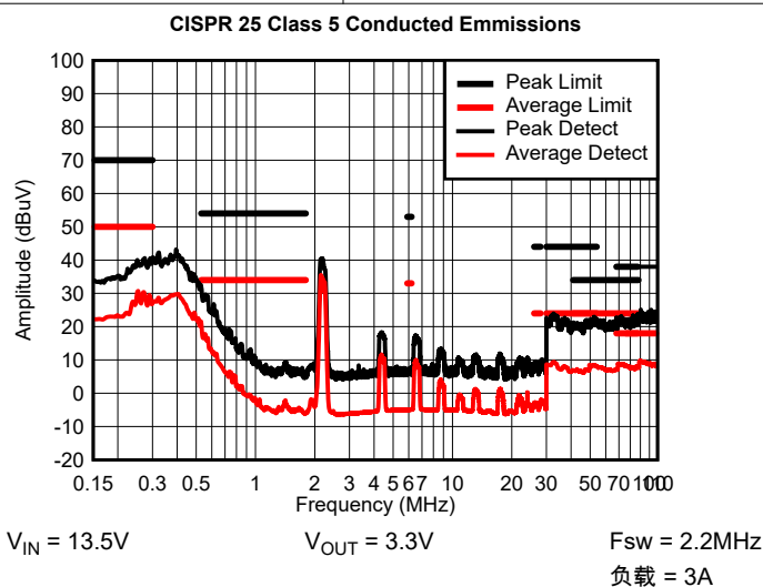
图 8-18. CISPR 25 5 类传导性 EMI 150kHz 至 108MHz 黑色：峰值检测，红色：平均值检测
