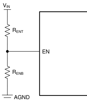
图 7-1. 使用 EN 引脚时的 VIN UVLO
