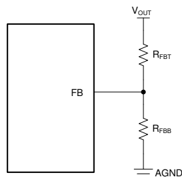
图 7-8. 为可调输出选项设置输出电压
