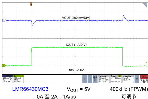
图 8-24. 负载瞬态
