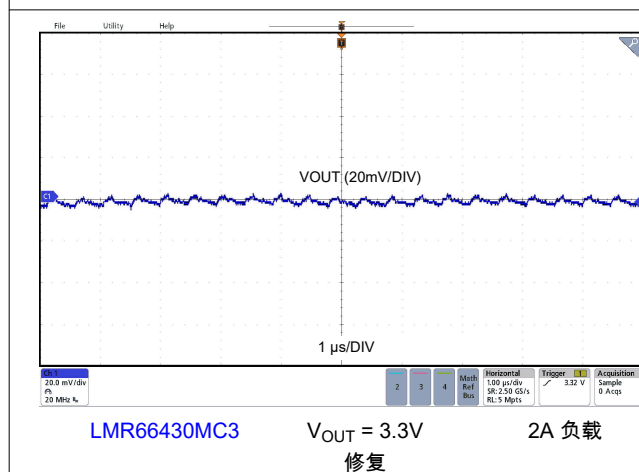
图 8-14. 输出电压纹波
