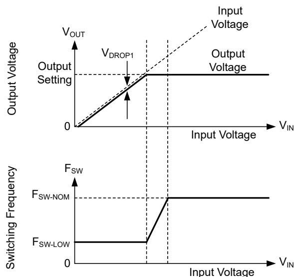
图 7-20. 压降中的频率和输出电压
