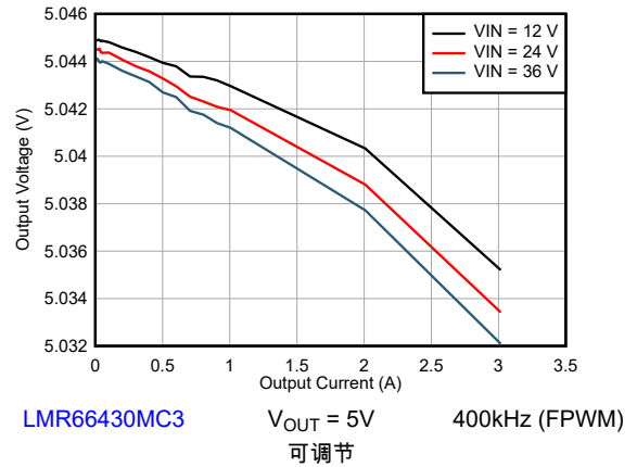
图 8-21. 线性 and 负载调整率
