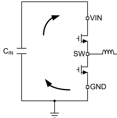
图 8-26. 具有快速边沿的电流环路
