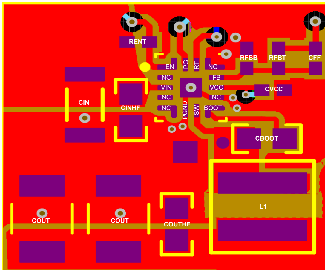
图 8-27. 布局示例
