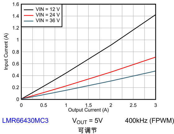
图 8-22. 输入电流与负载电流间的关系
