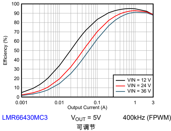
图 8-20. 效率
