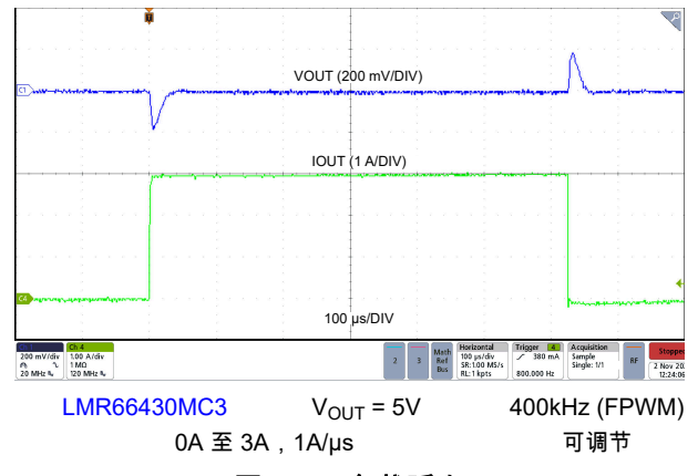
图 8-23. 负载瞬态
