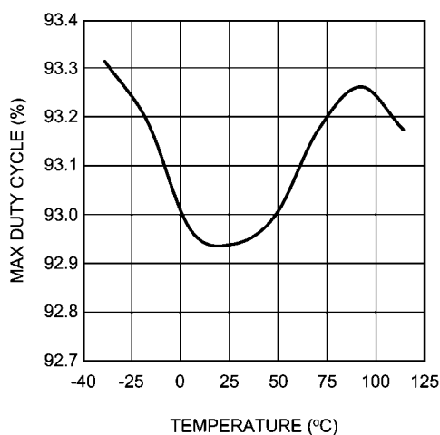
最大占空比与温度的关系曲线
