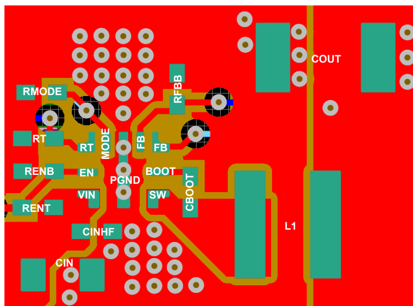
图 8-13. 固定输出版本
