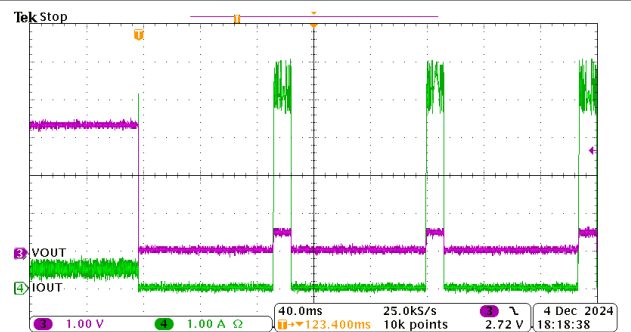
器件类型 = 4A 3.3V 固定输出 模式 = FPWM F_{SW} = 2\text{MHz}
