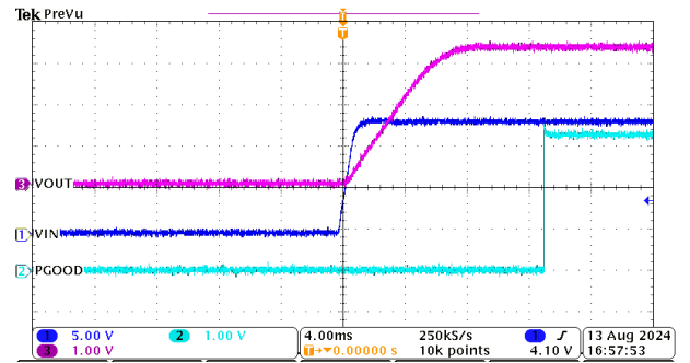
器件类型 = 4A 3.3V 固定输出 模式 = AUTO F_{SW} = 2\text{MHz}
