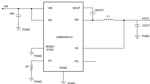
简化版原理图 - 固定输出
