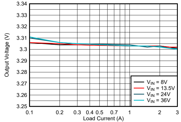
图 8-3. 负载调整率
