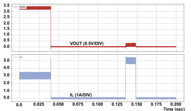
图 8-9. 应用短路
