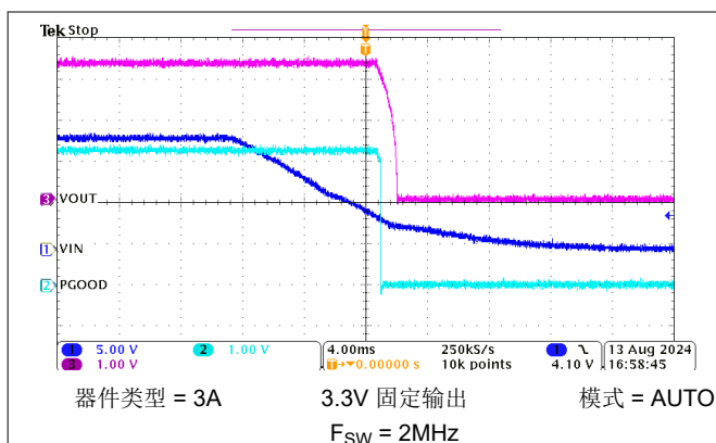
图 8-8. 关断操作
