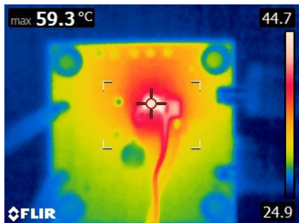
图 8-9. 应用短路
