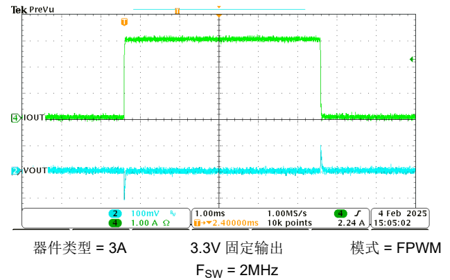
图 8-5. 20mA 至 3A 负载瞬态
