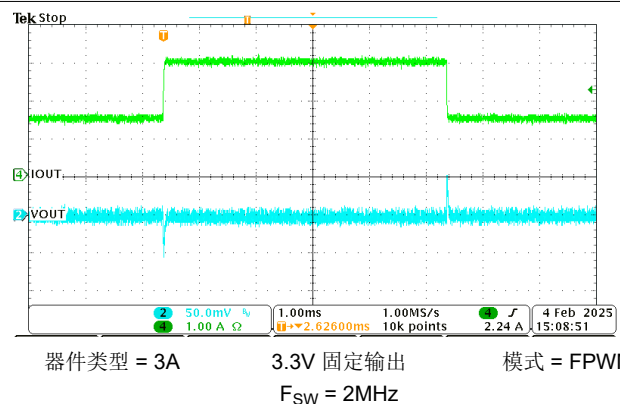
图 8-6. 1.5A 至 3A 负载瞬态
