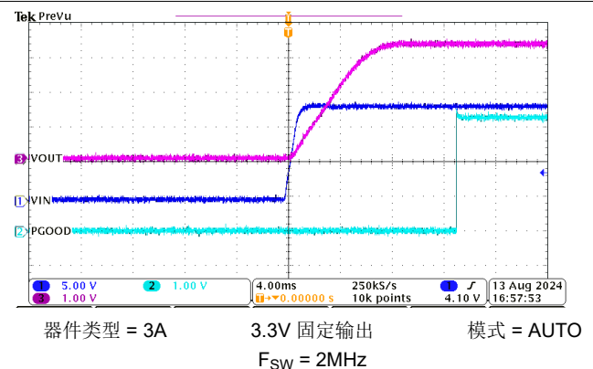
图 8-7. 启动运行
