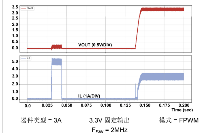
图 8-10. 短路恢复
