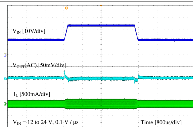
图 8-8. Line Transient
