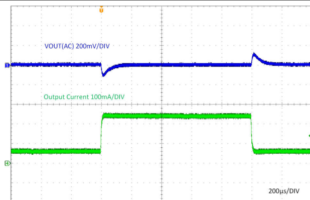
图 8-7. 负载瞬态 (60mA 至 240mA)
