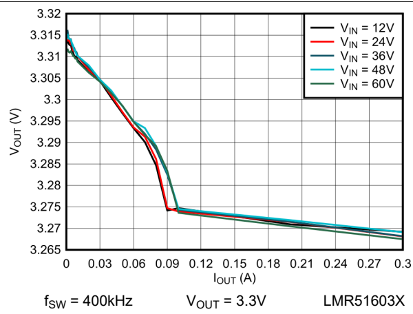
图 6-10. 负载调整 (3.3V)
