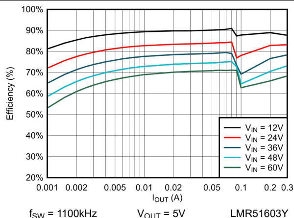
图 6-1. PFM 效率与负载电流间的关系 (5V)
