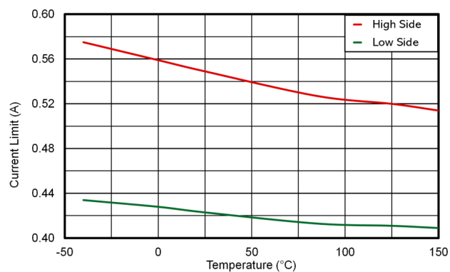
图 6-14. HS 和 LS 电流限制与温度间的关系
