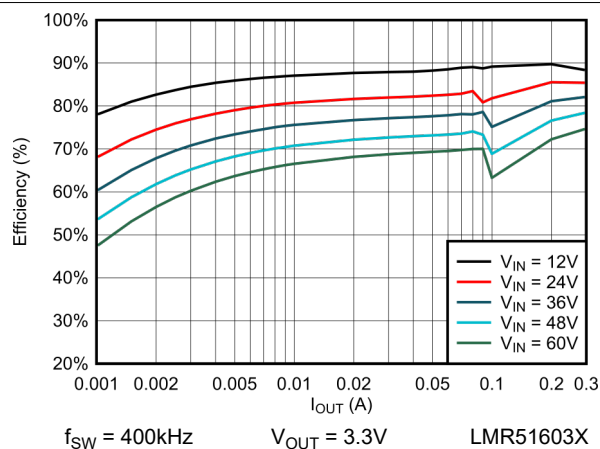
图 6-5. PFM 效率与负载电流间的关系 (3.3V)
