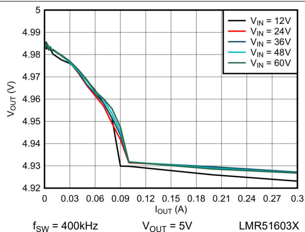
图 6-9. 负载调整 (5V)
