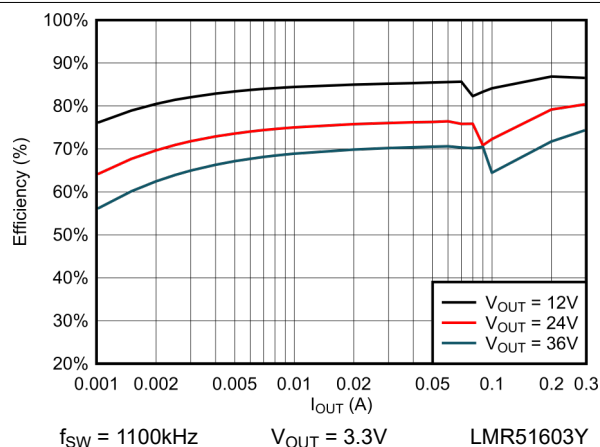
图 6-3. PFM 效率与负载电流间的关系 (3.3V)
