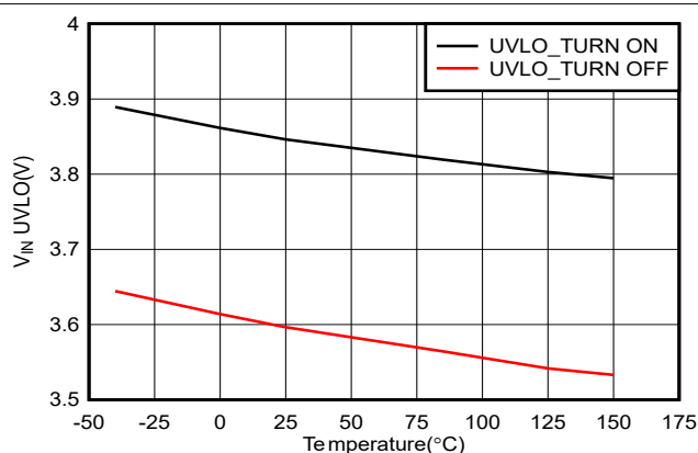
图 6-12. V_{IN} UVLO 与温度间的关系
