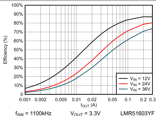
图 6-4. FPWM 效率与负载电流间的关系 (3.3V)
