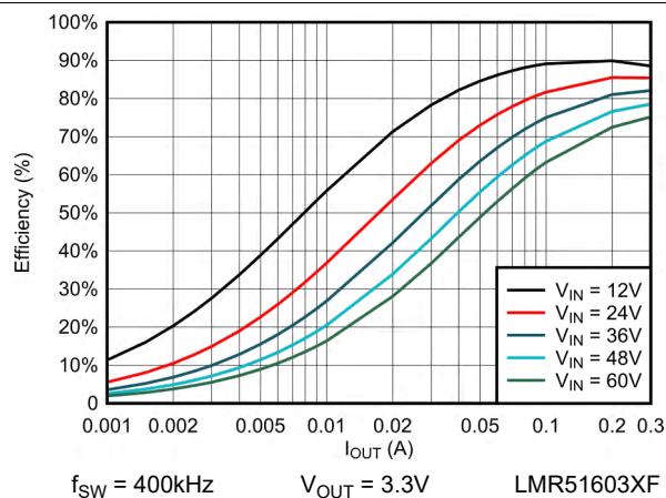
图 6-6. FPWM 效率与负载电流间的关系 (3.3V)
