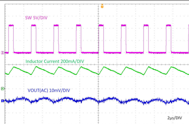
图 8-4. 满载时的纹波
