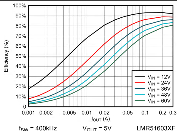
图 6-8. FPWM 效率与负载电流间的关系 (5V)
