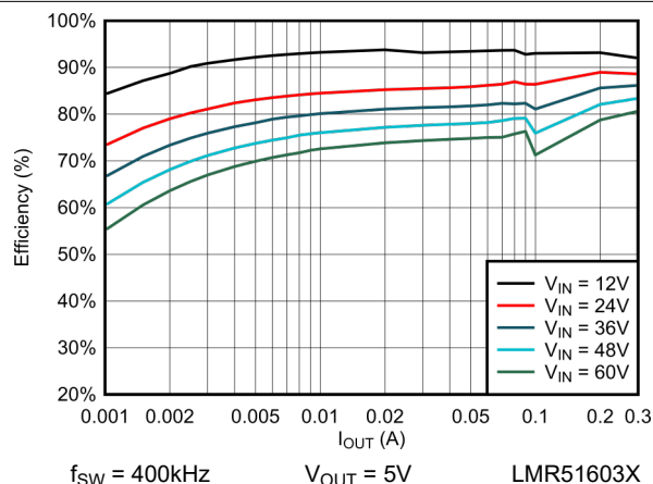
图 6-7. PFM 效率与负载电流间的关系 (5V)
