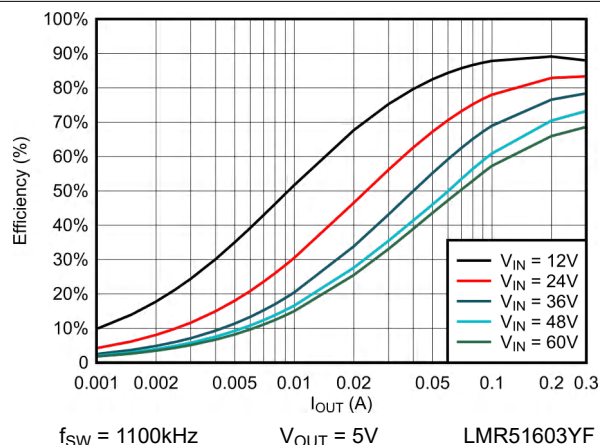
图 6-2. FPWM 效率与负载电流间的关系 (5V)
