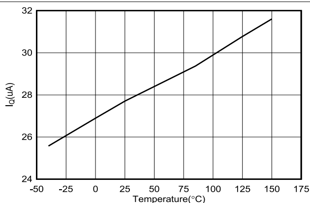
图 6-11. V_{IN} 静态电流与温度间的关系
