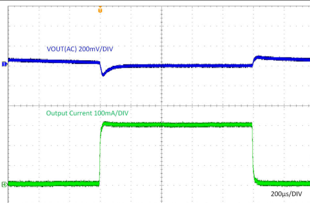
图 8-8. 负载瞬态 (0mA 至 300mA)
