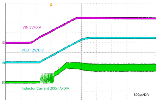
图 8-5. 由 V_{IN} 启动
