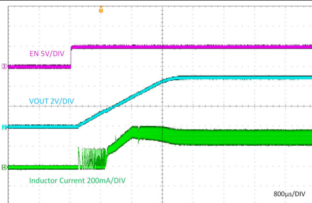
图 8-6. 由 EN 启动
