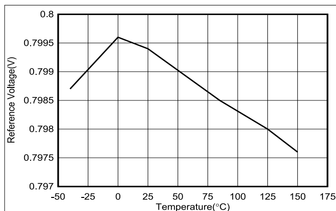
图 6-13. 基准电压与温度间的关系
