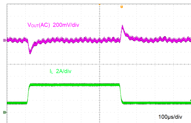
图 8-6. 负载瞬态
