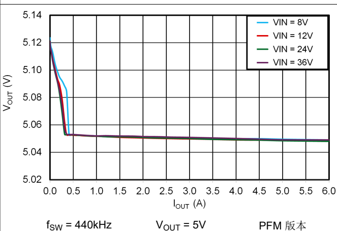
图 6-4. 5V 负载调整
