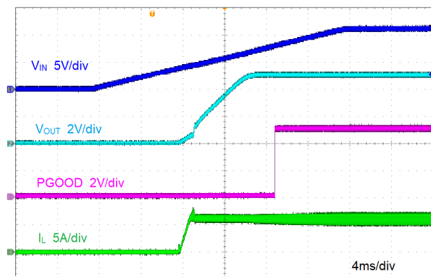
图 8-4. 由 V_{IN} 启动
