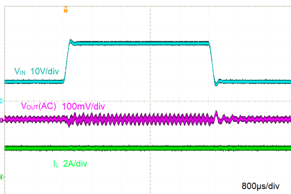
图 8-7. 线路瞬态
