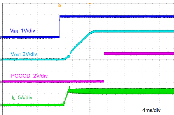
图 8-5. 由 EN 启动
