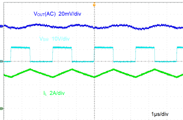
图 8-3. 满载时的纹波
