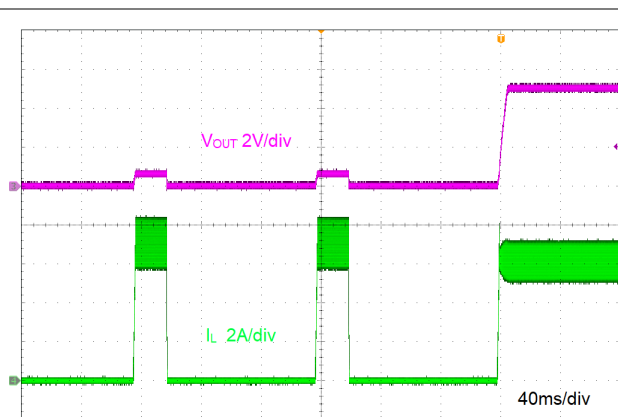
图 8-9. 短路恢复
