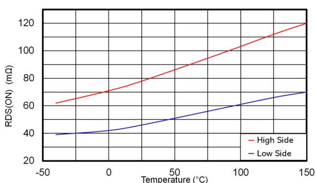
图 7-12. 高侧和低侧开关 R_{DS(on)}
