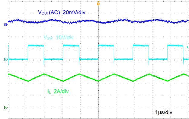
图 9-3. 满载时的纹波
