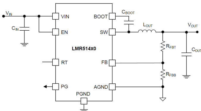
简化原理图
