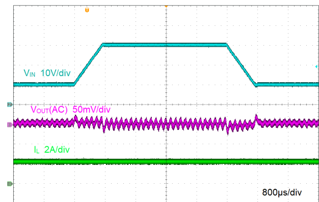
图 9-7. 线路瞬态
