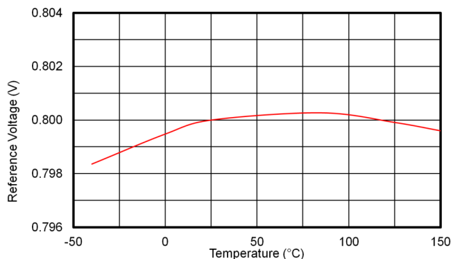
图 7-11. 基准电压
