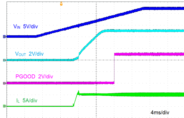
图 9-4. 由 V_{IN} 启动
