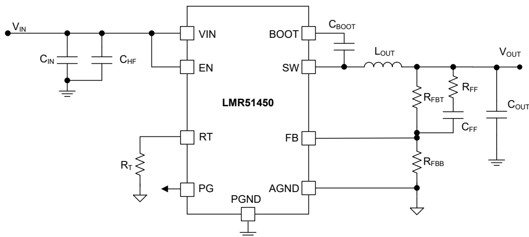
图 9-1. 应用电路
