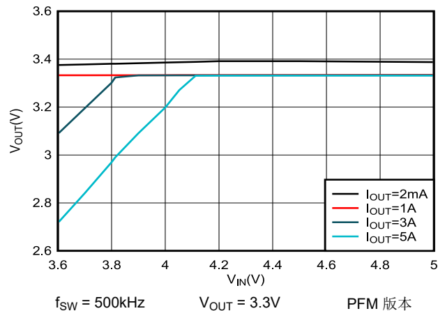
图 7-8. 3.3V 压降
