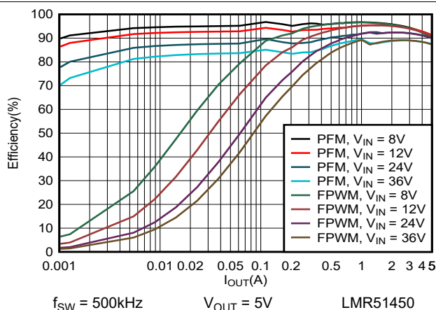
图 7-1. 5V 效率与负载电流间的关系
