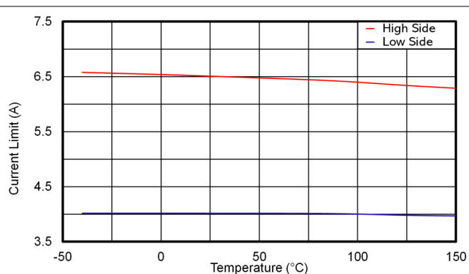
图 7-14. LMR51440 高侧和低侧电流限值
