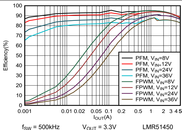
图 7-3. 3.3V 效率与负载电流间的关系
