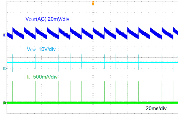
图 9-2. 空载时的纹波
