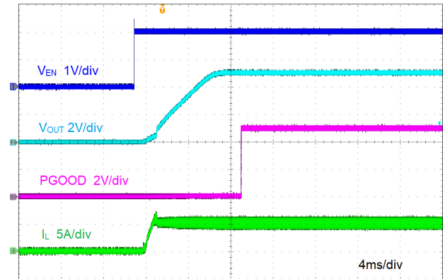
图 9-5. 由 EN 启动
