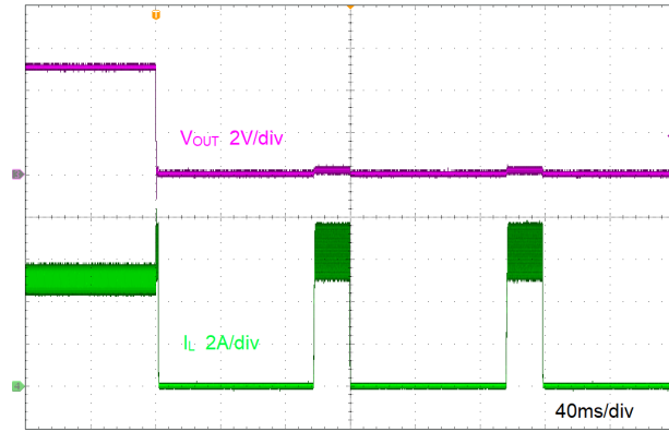
图 9-8. 短路保护
