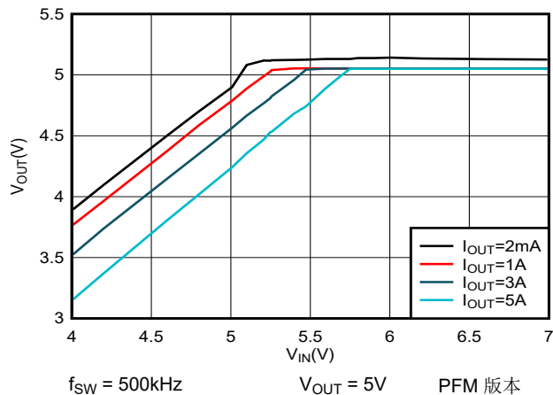
图 7-7. 5V 压降
