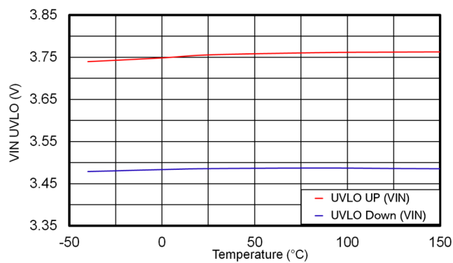
图 7-10. VIN UVLO
