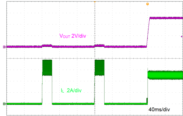
图 9-9. 短路恢复
