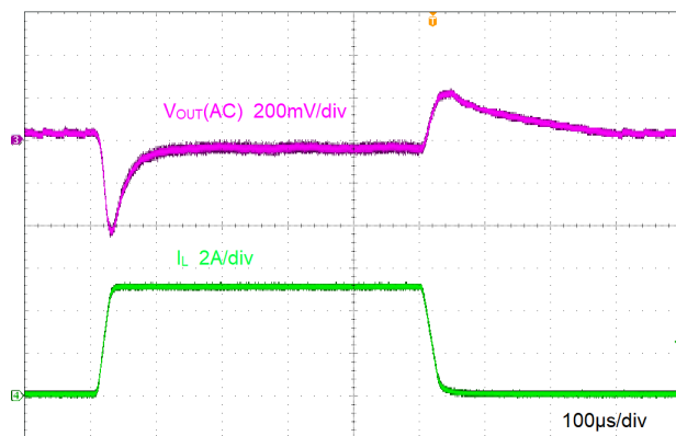
图 9-6. 负载瞬态
