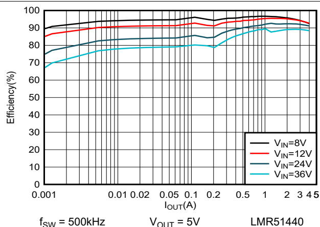
图 7-2. 5V 效率与负载电流间的关系
