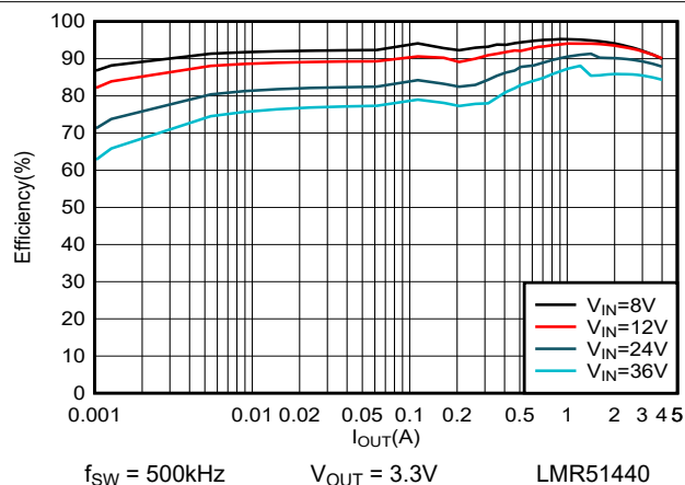
图 7-4. 3.3V 效率与负载电流间的关系
