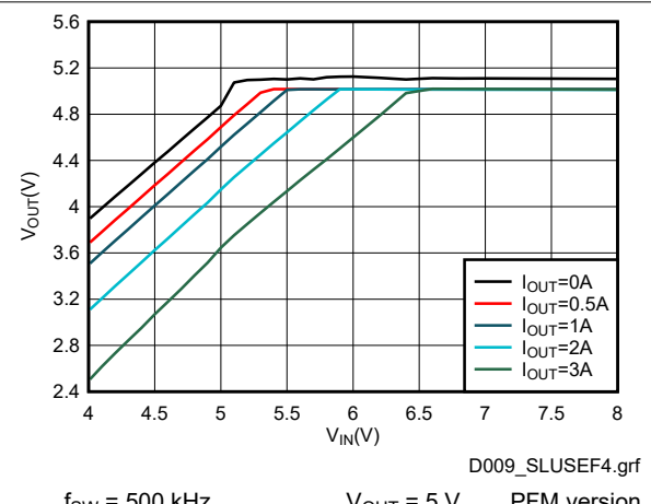
图 7-6. 5-V Dropout
