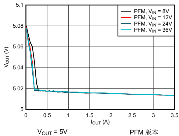
图 6-9. 5V 负载调整率
