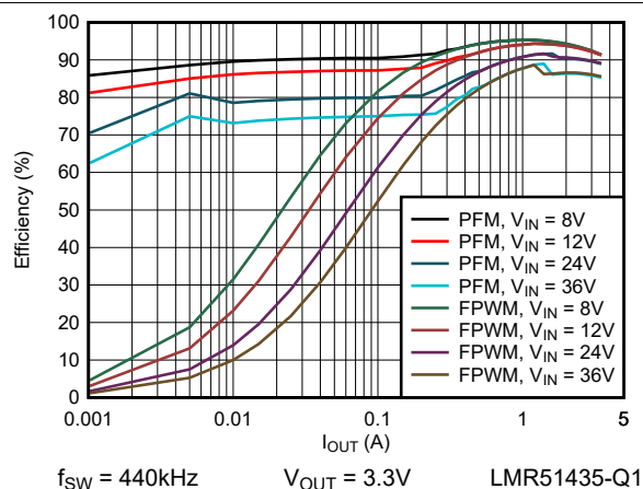
图 6-3. 3.3V 效率与负载电流间的关系
