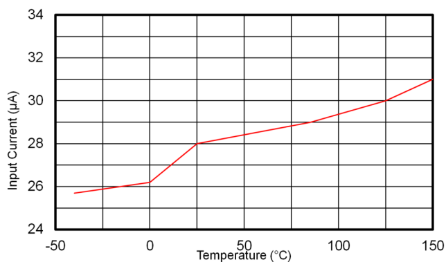
图 6-13. 非开关输入电源电流
