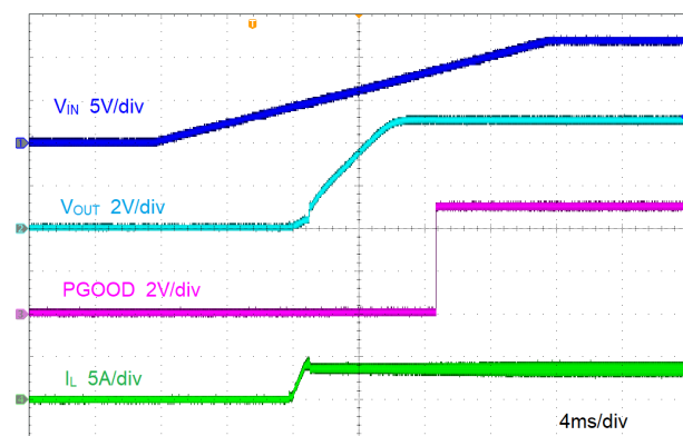
图 8-4. 由 V_{IN} 启动
