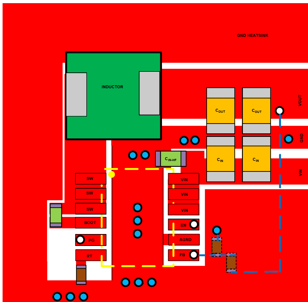
图 8-10. 布局
