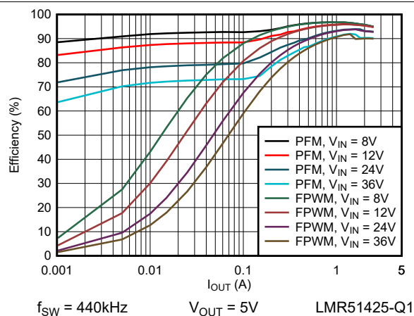
图 6-5. 5V 效率与负载电流间的关系
