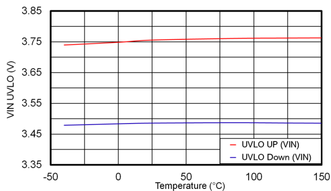
图 6-14. V_{IN} UVLO
