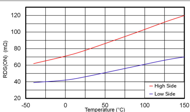
图 6-16. 高侧和低侧开关 R_{DS(on)}
