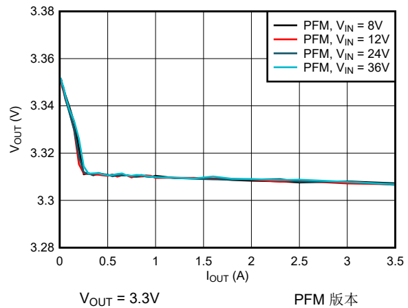
图 6-10. 3.3V 负载调整率
