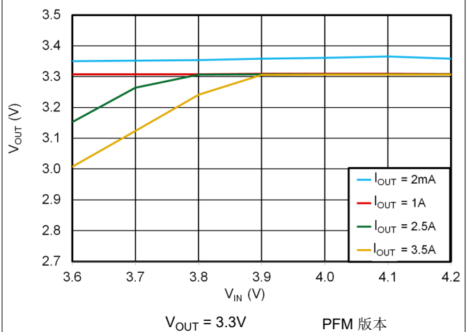
图 6-12. 3.3V 压降
