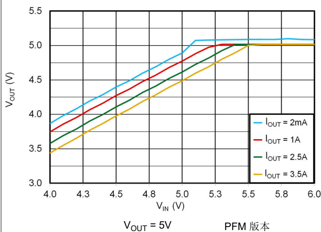
图 6-11. 5V 压降
