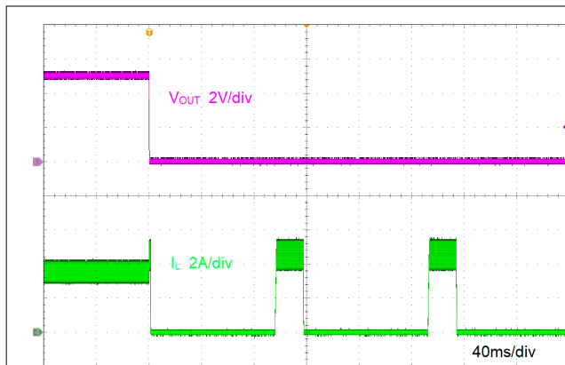
图 8-8. 短路保护
