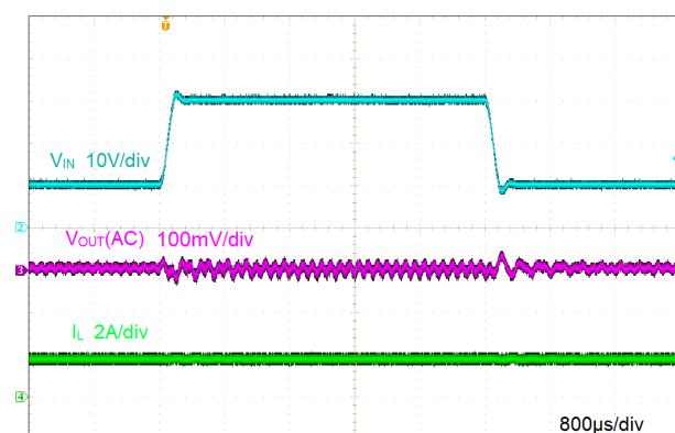
图 8-7. 线路瞬态
