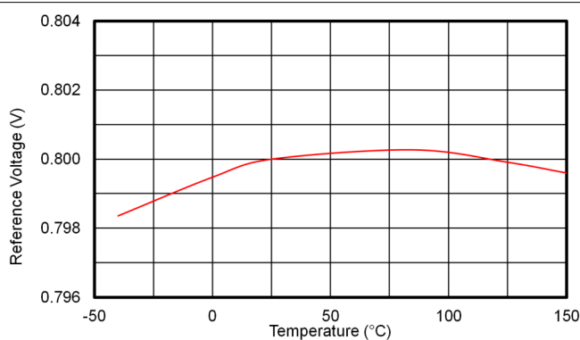
图 6-15. 基准电压
