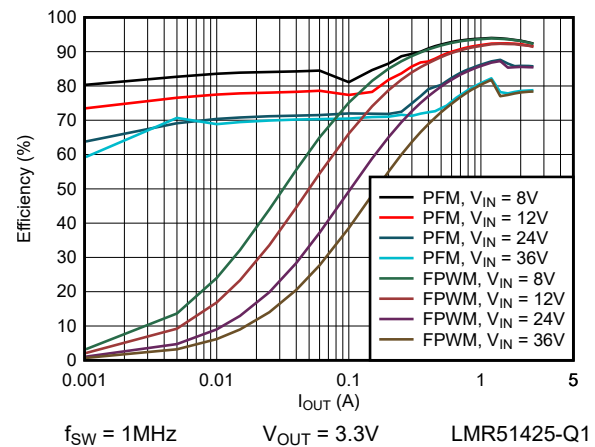
图 6-8. 3.3V 效率与负载电流间的关系
