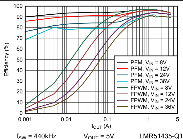
图 6-1. 5V 效率与负载电流间的关系
