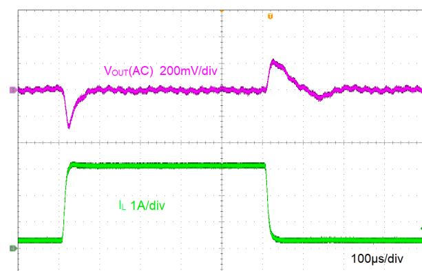
图 8-6. 负载瞬态
