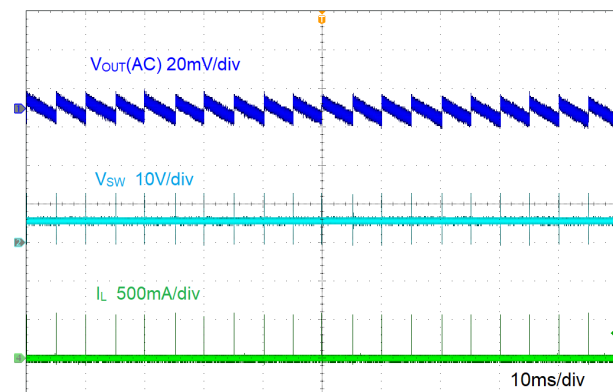
图 8-2. 空载时的纹波
