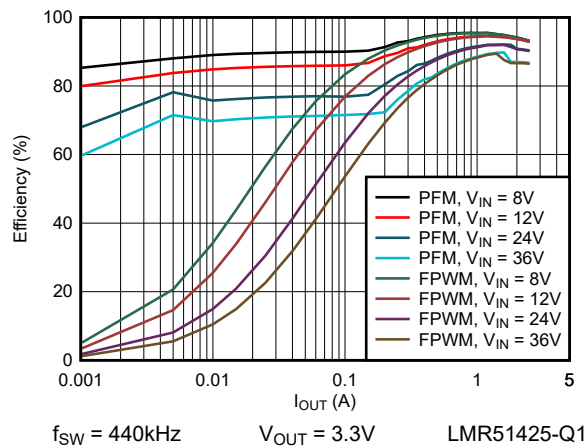
图 6-7. 3.3V 效率与负载电流间的关系
