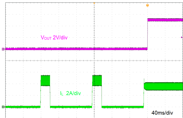
图 8-9. 短路恢复
