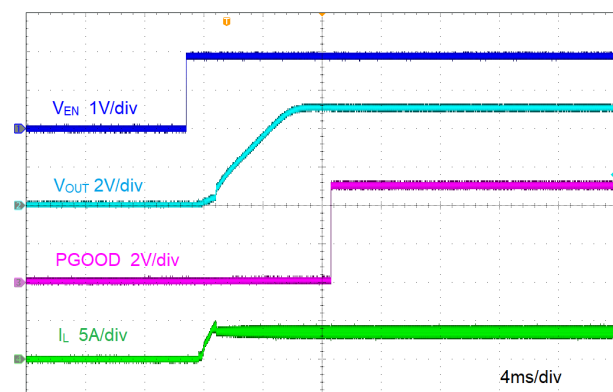
图 8-5. 由 EN 启动
