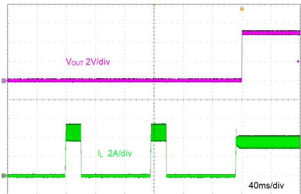
图 8-9. 短路恢复
