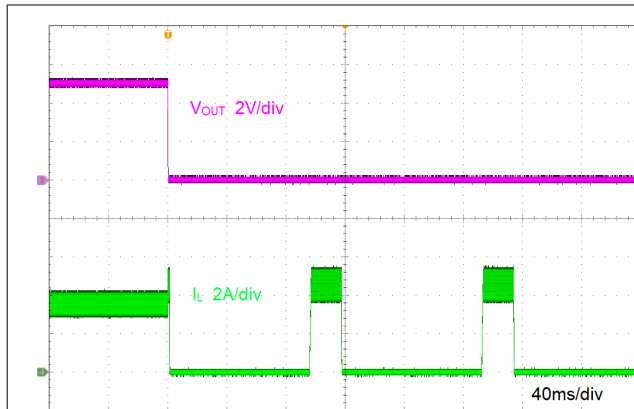
图 8-8. 短路保护
