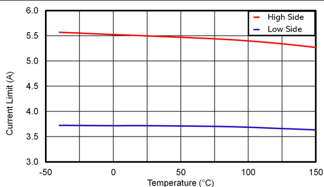
图 6-17. LMR51435 高侧和低侧电流限值
