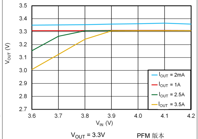
图 6-12. 3.3V 压降
