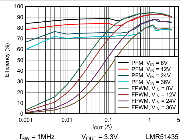
图 6-4. 3.3V 效率与负载电流间的关系
