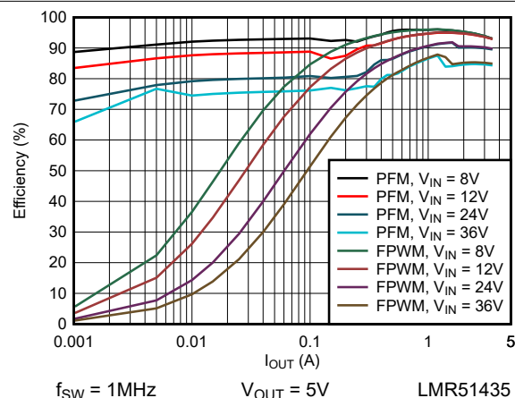
图 6-2. 5V 效率与负载电流间的关系
