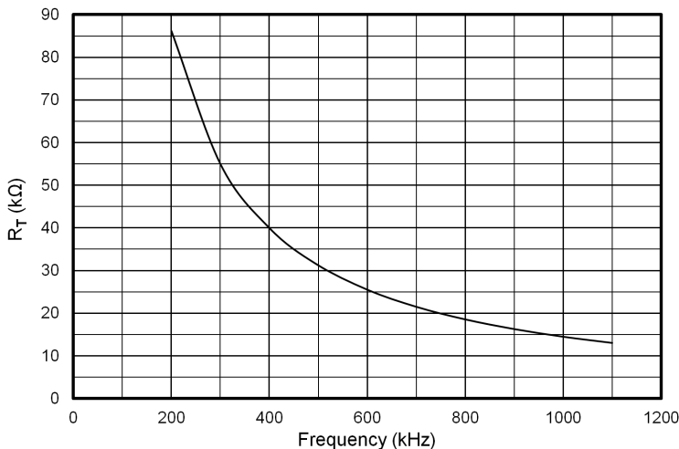
图 7-4. R_T 与频率曲线间的关系
