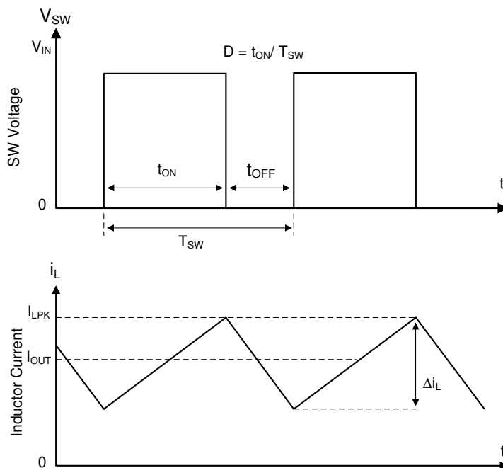
图 7-1. 连续导通模式 (CCM) 下的 SW 节点和电感器电流波形
