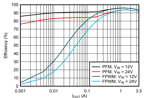
效率与输出电流间的关系， V_{OUT} = 5V ，500kHz
