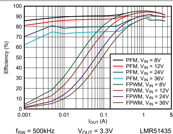
图 6-3. 3.3V 效率与负载电流间的关系
