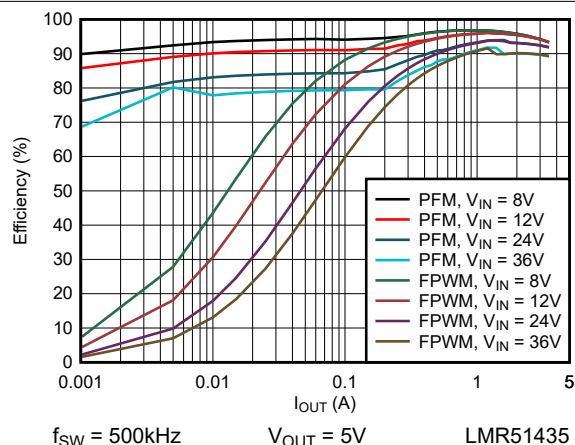
图 6-1. 5V 效率与负载电流间的关系
