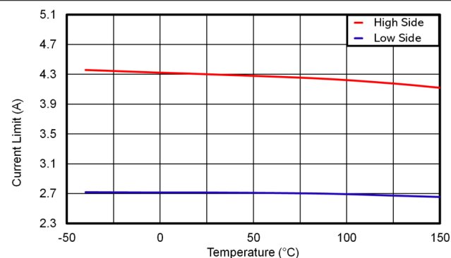
图 6-18. LMR51425 高侧和低侧电流限值
