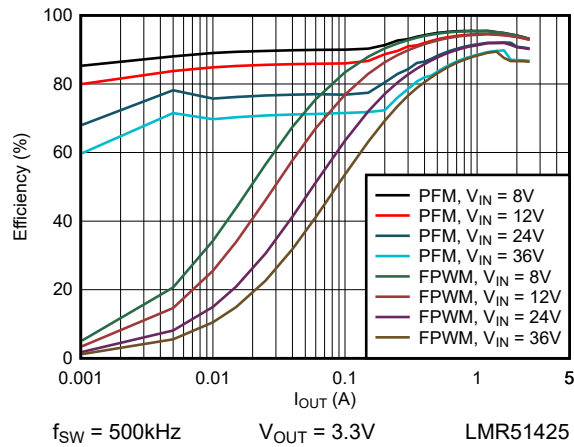
图 6-7. 3.3V 效率与负载电流间的关系
