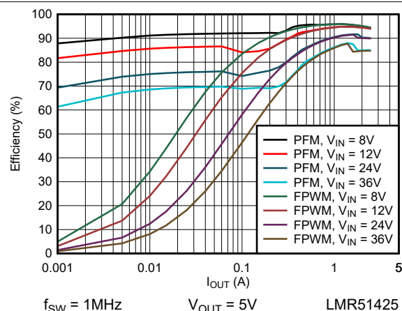
图 6-6. 5V 效率与负载电流间的关系
