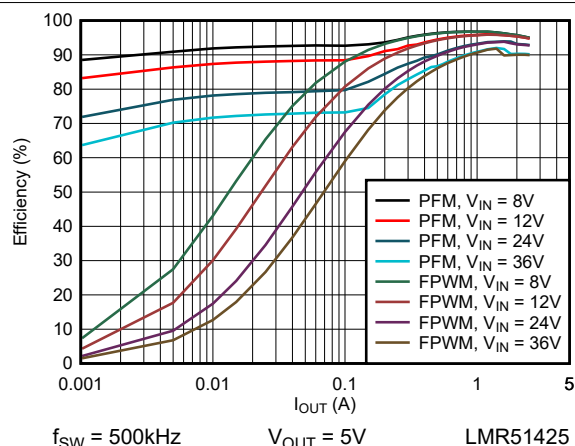
图 6-5. 5V 效率与负载电流间的关系
