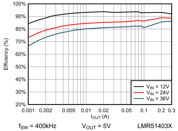
图 6-2. 效率与负载电流间的关系 (5V)
