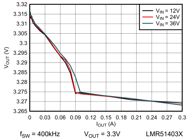
图 6-6. 负载调整率 (3.3V)
