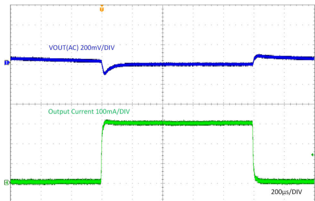
图 8-8. 负载瞬态 (0mA 至 300mA)
