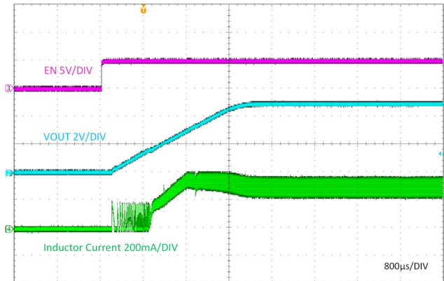
图 8-6. 由 EN 启动
