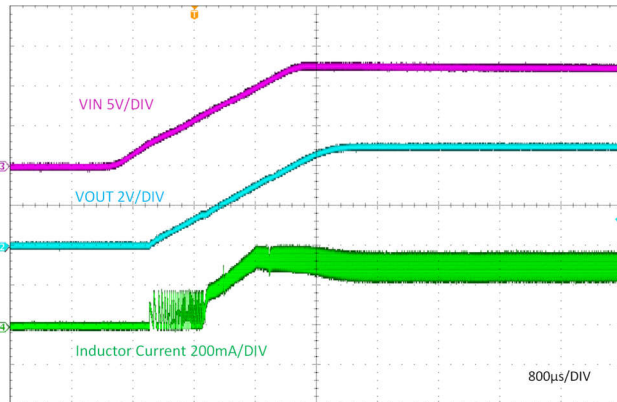
图 8-5. 由 V_{IN} 启动
