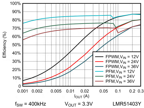
图 6-3. 效率与负载电流间的关系 (3.3V)
