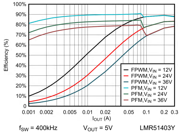
图 6-4. 效率与负载电流间的关系 (5V)
