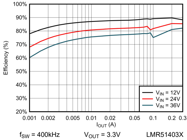
图 6-1. 效率与负载电流间的关系 (3.3V)
