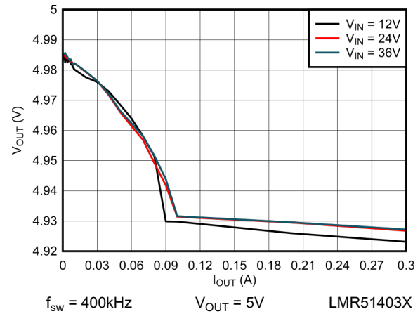
图 6-5. 5V 时的负载调整
