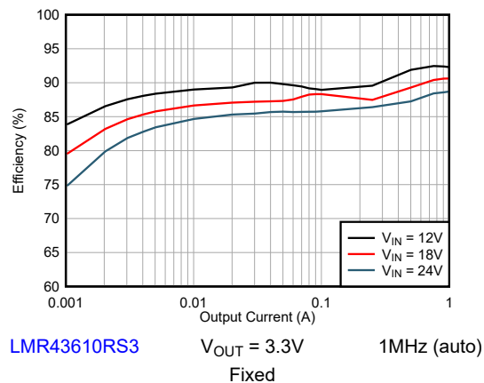
图 8-7. Efficiency
