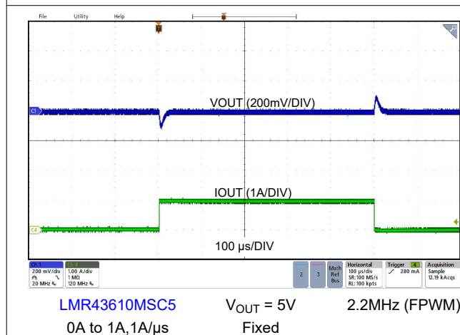
图 8-19. Load Transient
