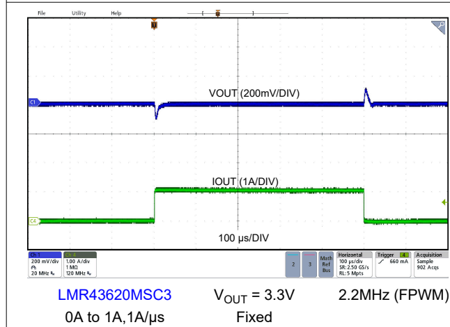
图 8-17. Load Transient
