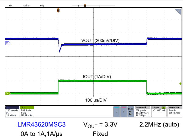
图 8-18. Load Transient
