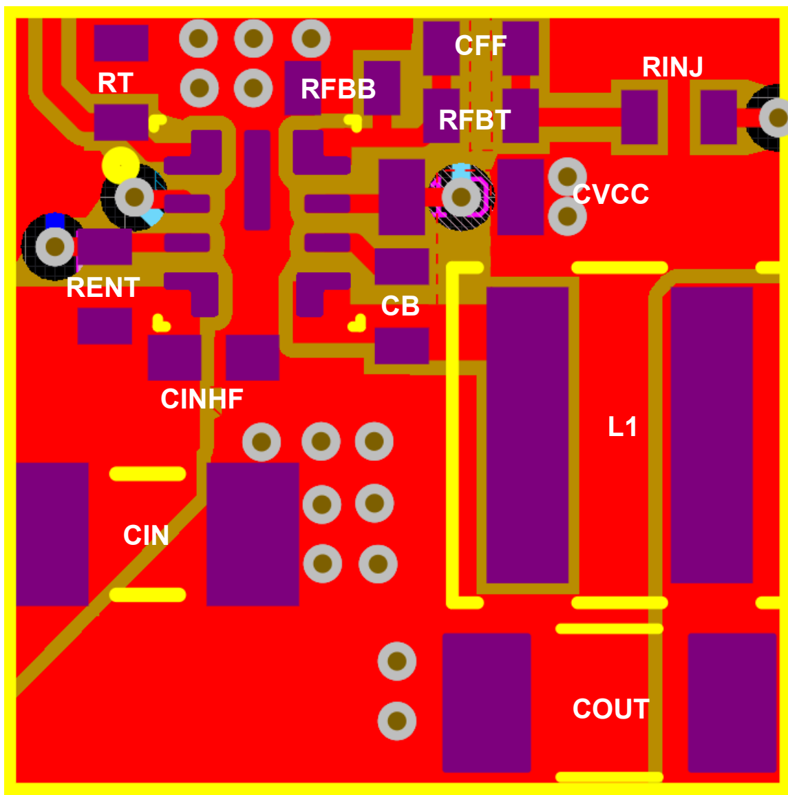
图 8-32. Example Layout
