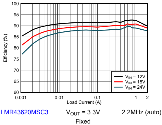
图 8-3. Efficiency
