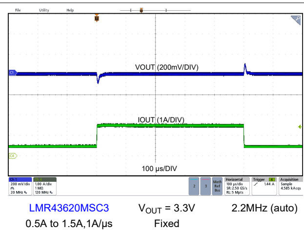
图 8-16. Load Transient
