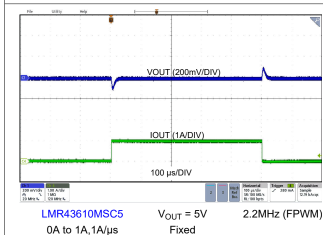
图 8-19. Load Transient
