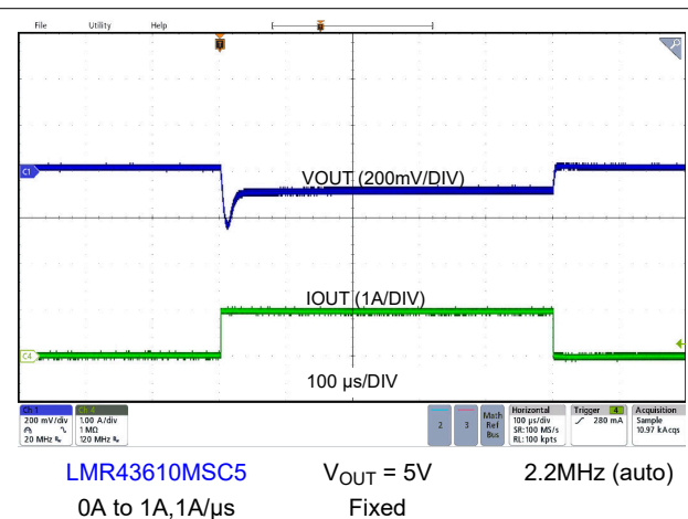
图 8-20. Load Transient
