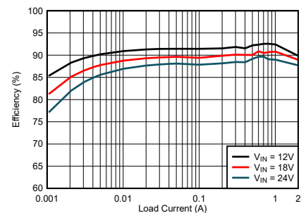
效率： V_{\text{OUT}} = 3.3\text{V} (固定值)、 2.2\text{MHz}
