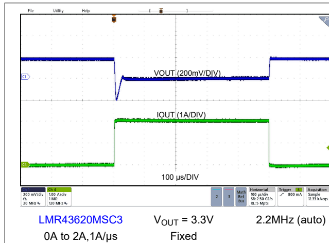
图 8-15. Load Transient
