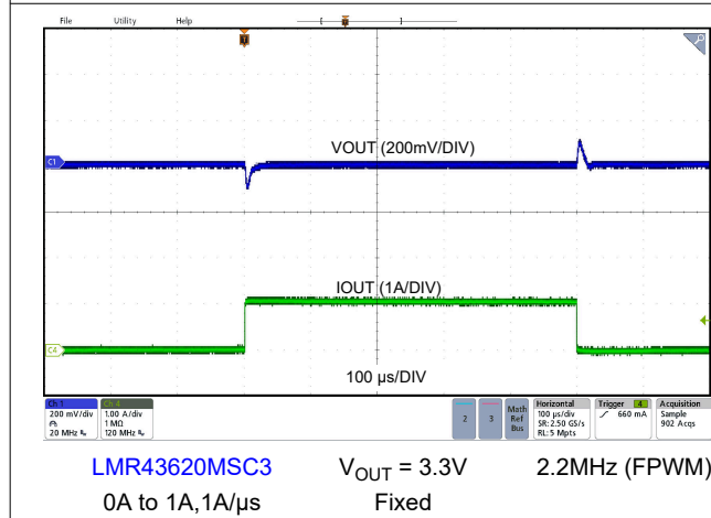
图 8-17. Load Transient
