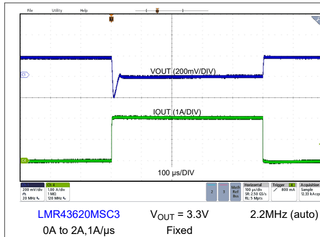
图 8-15. Load Transient
