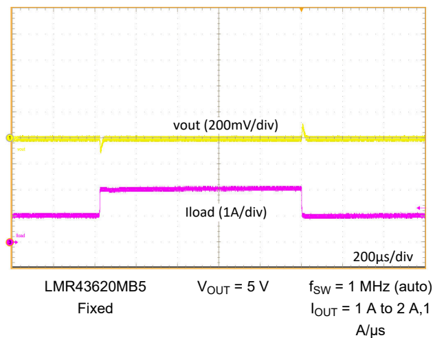
图 9-9. Load Transient
