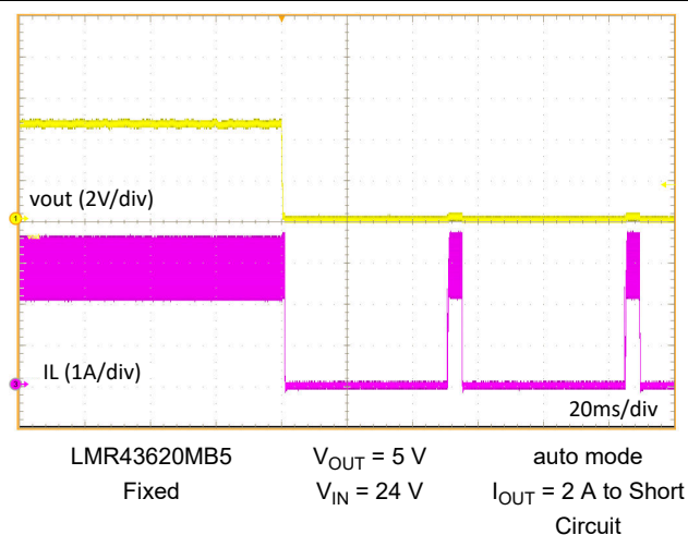
图 9-11. Short-Circuit Protection
