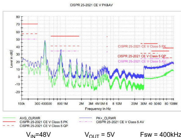
图 8-15. 典型的 CISPR 25 传导 EMI 150kHz 至 108MHz 绿色：平均值检测，蓝色 = 峰值检测
