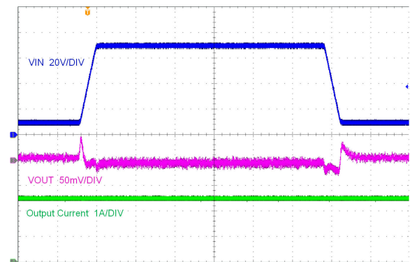
LMR38025-Q1(PFM) V_{OUT} = 5V 400kHz ( 交流耦合 ) 800μs/DIV 200V/ms 时为 10V 至 70V
