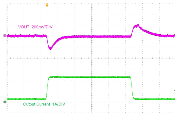
LMR38025-Q1(PFM) V_{OUT} = 5V 400kHz , ( 交流耦合 ) 100μs/DIV 200mA/μs 时为 250mA 至 2.25A
