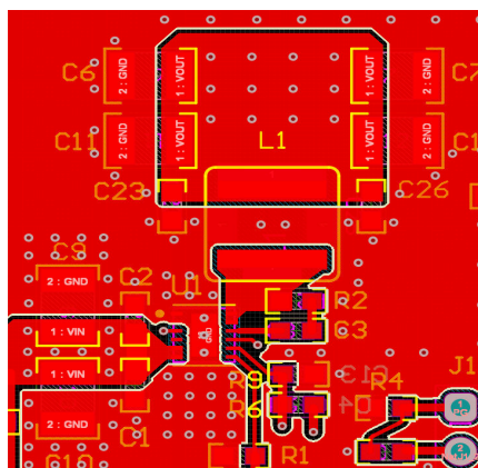
图 8-18. WSON (DRR) 封装的布局示例
