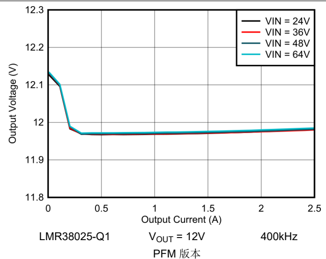
图 8-14. 12V 负载调节
