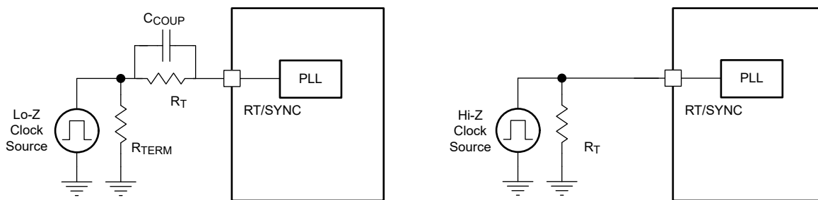
图 7-5. 与外部时钟同步
