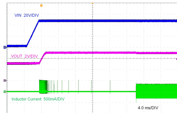
LMR38015-Q1 V_{OUT} = 5V 偏置为 3V 空载
