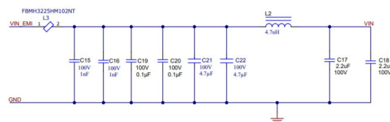
图 8-16. 典型 EMI 输入滤波器
