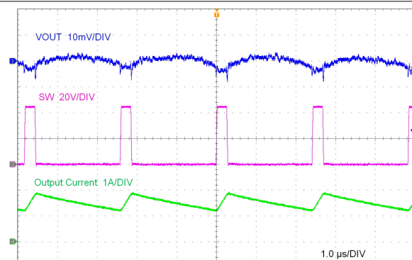
LMR38015-Q1 V_{OUT} = 5V 交流耦合 400kHz
