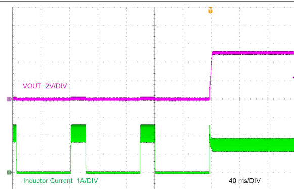
LMR38015-Q1 V_{OUT} = 5V 短路恢复
