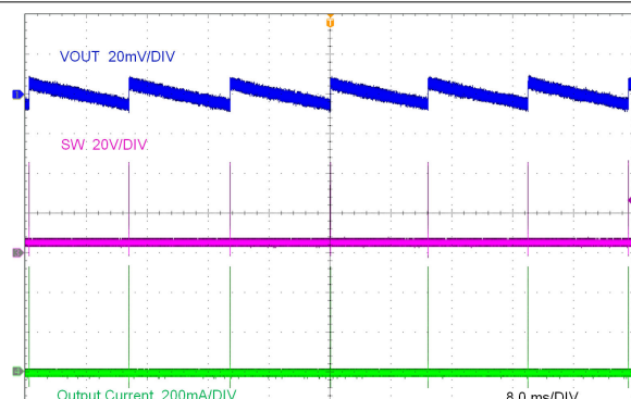
LMR38015-Q1 V_{OUT} = 5V 交流耦合 空载
