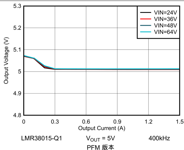
图 8-13. 5V 负载调整率
