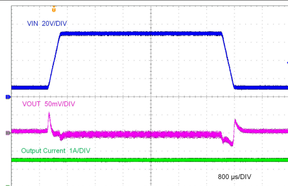
LMR38015-Q1 V_{OUT} = 5V (交流耦合) 400kHz 200V/ms 时为 10V 至 70V
