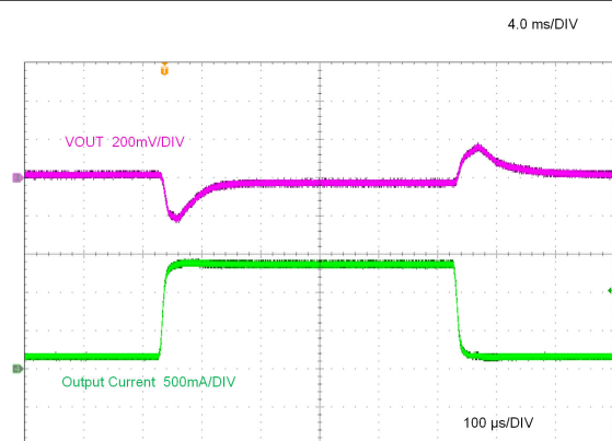
LMR38015-Q1 V_{OUT} = 5V (交流耦合) 400kHz 200mA/μs 时为 150mA 至 1350mA
