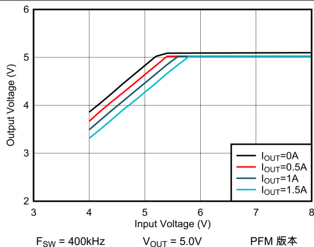
图 6-3. 5V 压降
