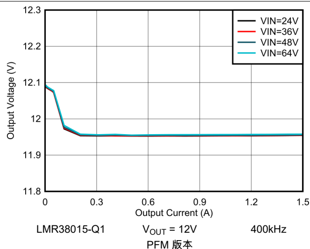
图 8-14. 12V 负载调整率
