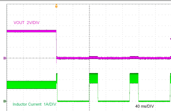
LMR38015-Q1 V_{OUT} = 5V 1A 到短路
