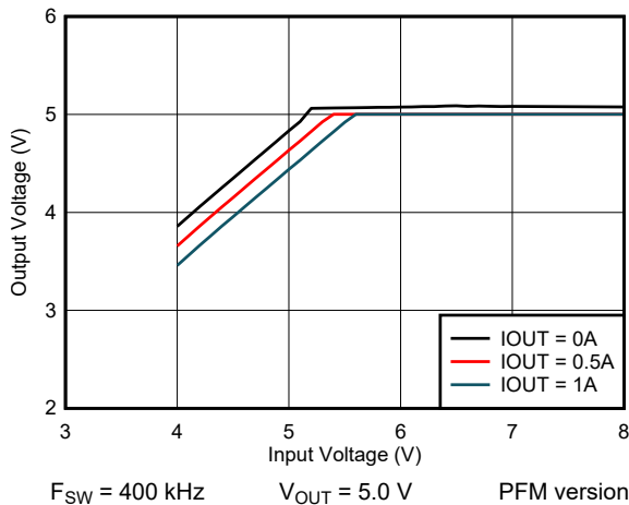
图 6-3. 5-V Dropout
