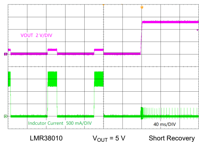
图 9-8. Short-Circuit Recovery
