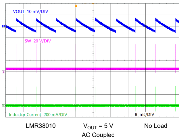
图 9-5. PFM Switching
