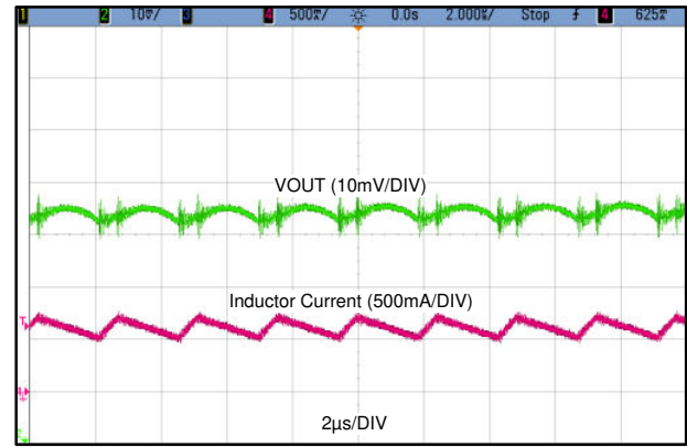
图 9-17. Output Ripple
