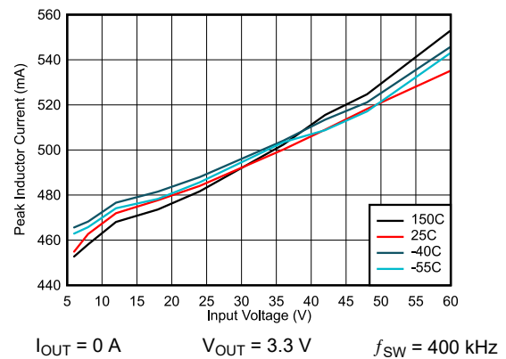
图 8-6. I_{PEAK-MIN}
