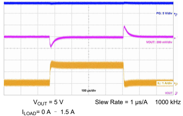
图 10-35. Load Transient
