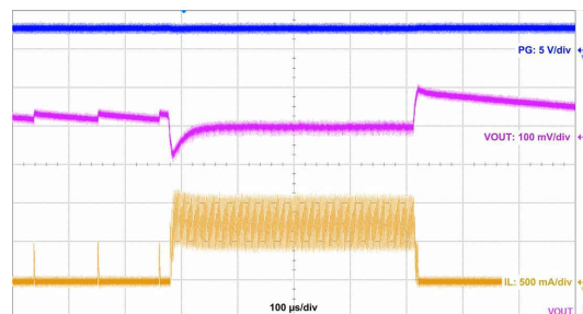
图 10-17. Load Transient
