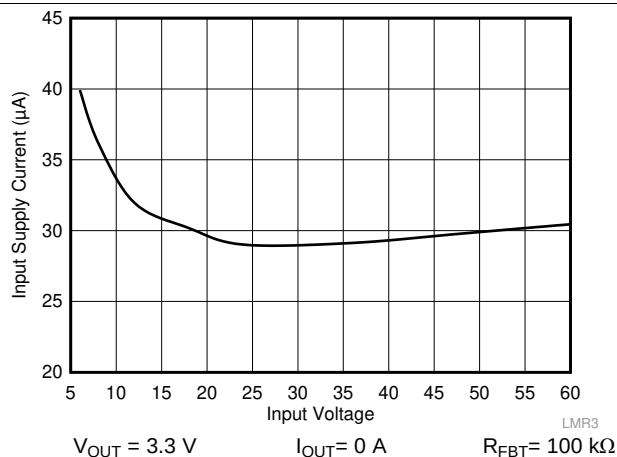
图 30. Input Supply Current
