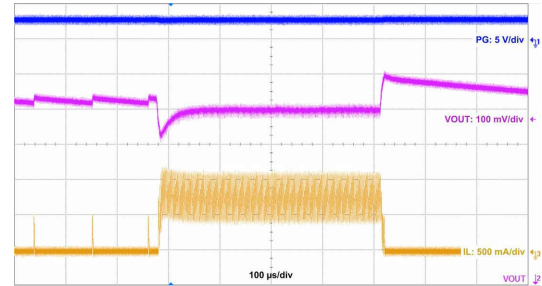
图 10-17. Load Transient
