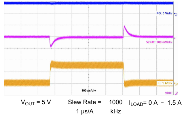
图 10-35. Load Transient
