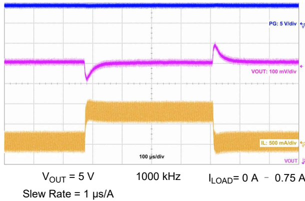
图 10-34. Load Transient
