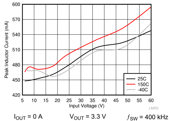
图 8-6. I_{PEAK-MIN}
