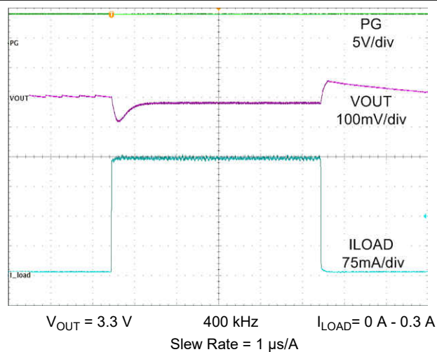
图 9-16. Load Transient
