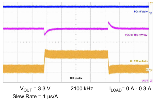
图 9-32. Load Transient
