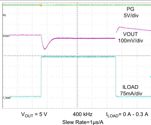
图 9-15. Load Transient
