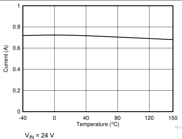
图 7-4. Low Side Current Limit
