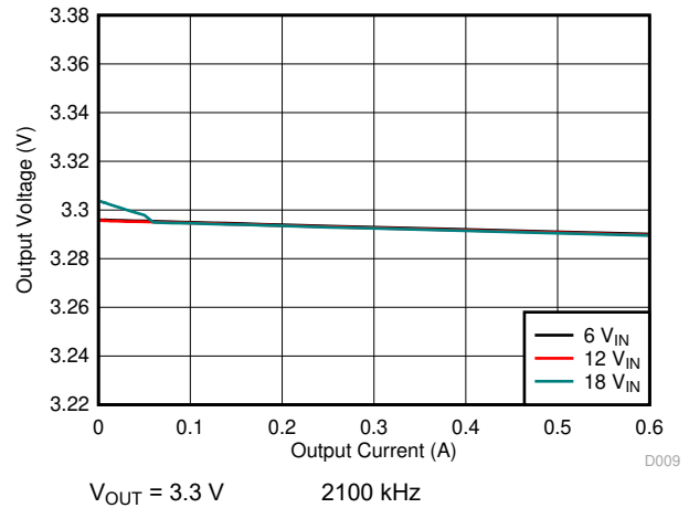
图 9-28. Load Regulation
