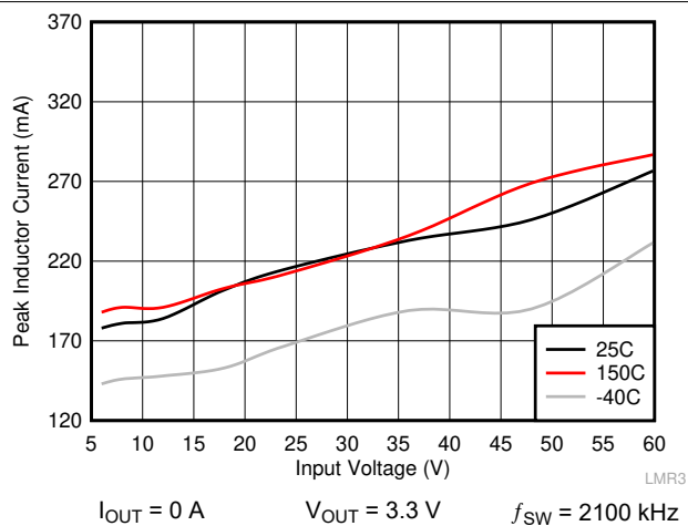
图 7-6. I_{PEAK-MIN}
