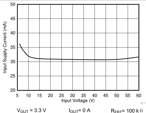
图 9-11. Input Supply Current
