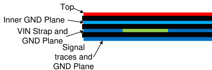
图 11-2. Example Layout
