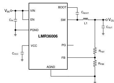
简化原理图
