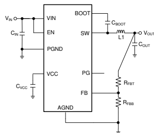
简化版原理图
