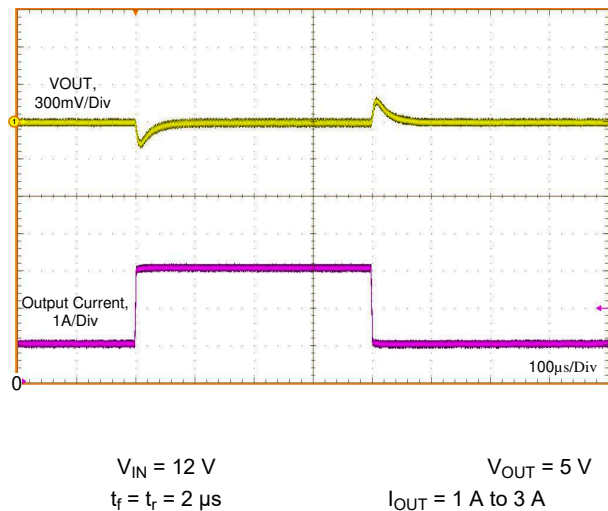
图 8-16. Load Transient
