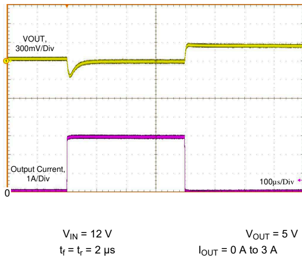
图 8-15. Load Transient
