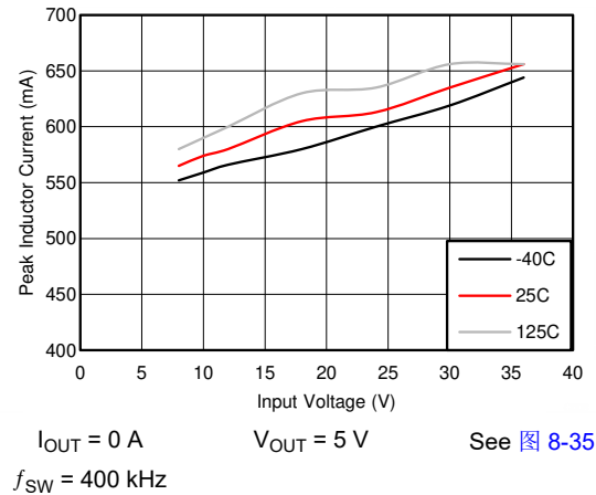
图 6-6. I_{PEAK-MIN}
