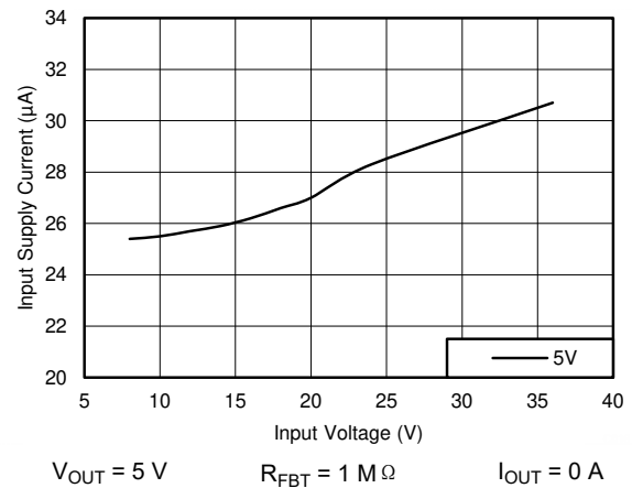
图 8-18. Input Supply Current
