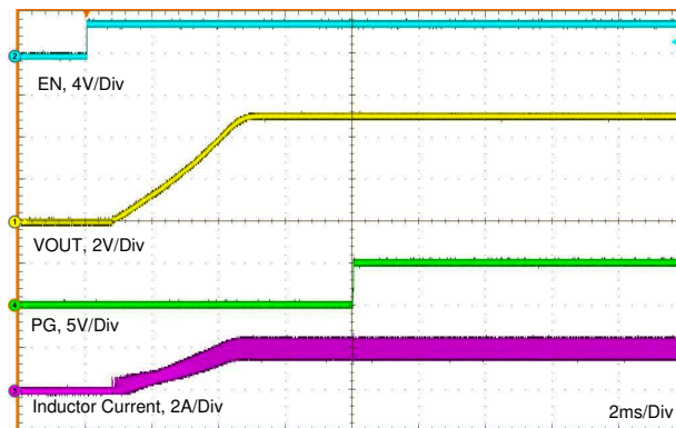
图 7-3. Precision Enable Behavior
