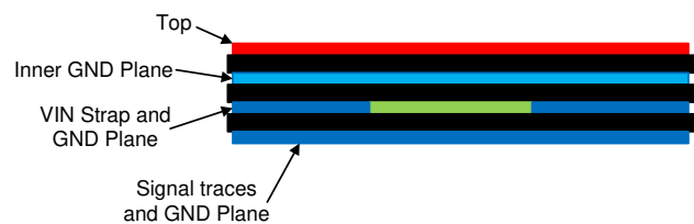
图 10-2. Example Layout for VQFN Package
