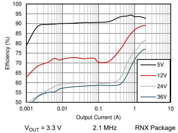
图 8-16. Efficiency
