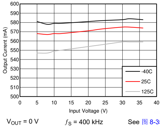
图 6-3. Short-Circuit Output Current
