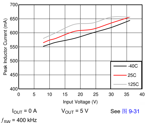
图 7-6. I_{PEAK-MIN}
