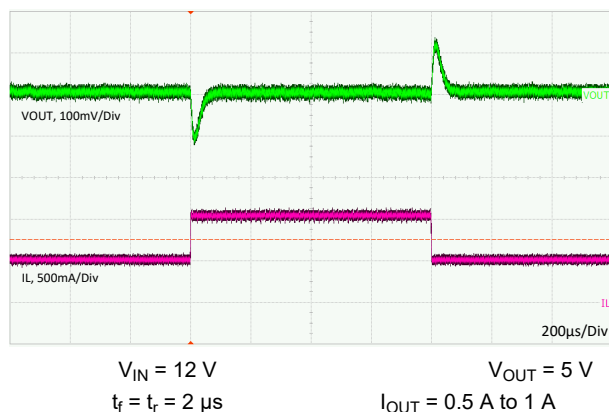
图 9-18. Load Transient
