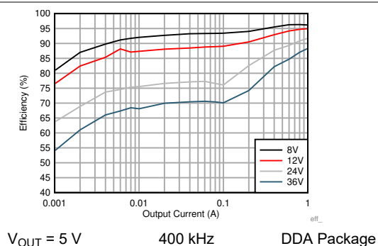
图 9-6. Efficiency
