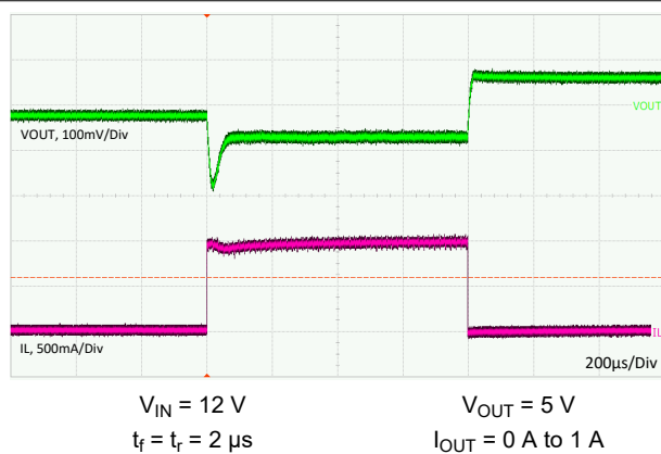
图 9-16. Load Transient
