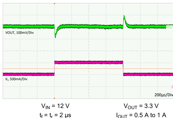
图 9-19. Load Transient
