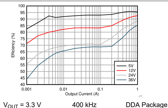
图 9-7. Efficiency
