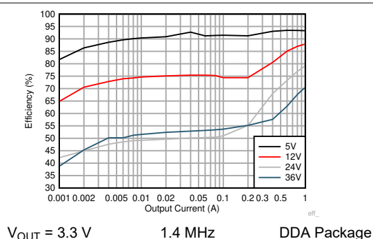
图 9-9. Efficiency
