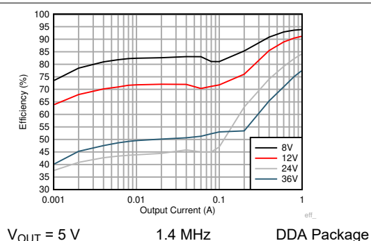
图 9-8. Efficiency
