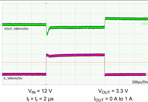
图 9-17. Load Transient
