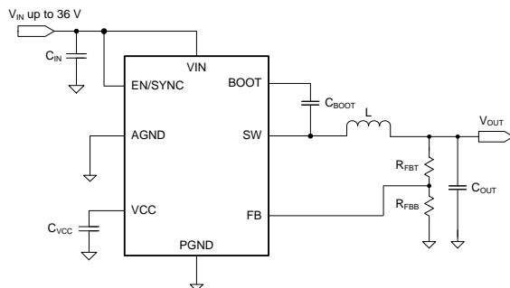
简化原理图
