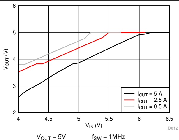
图 5-8. 压降曲线
