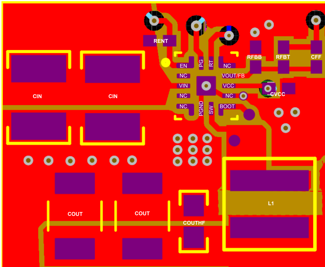
图 9-13. Example Layout
