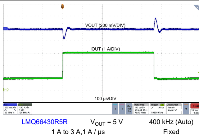
图 9-9. Load Transient
