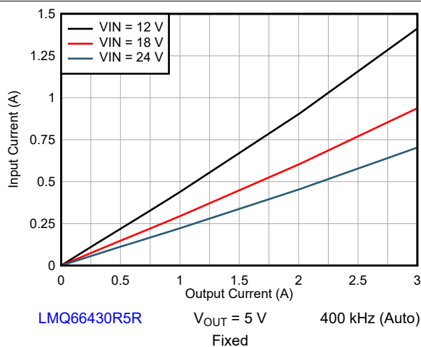
图 9-6. Input Current vs Load Current
