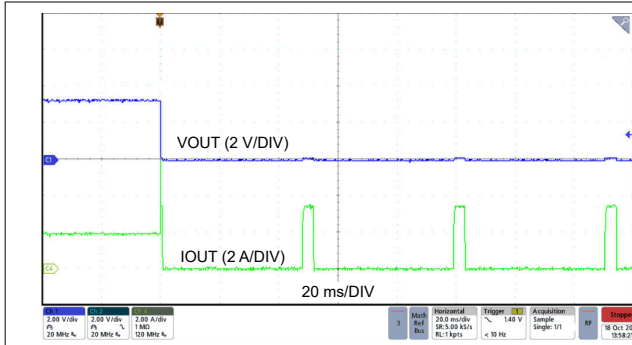
图 8-11. Hiccup Entry
