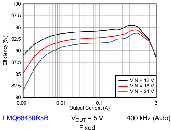
图 9-4. Efficiency
