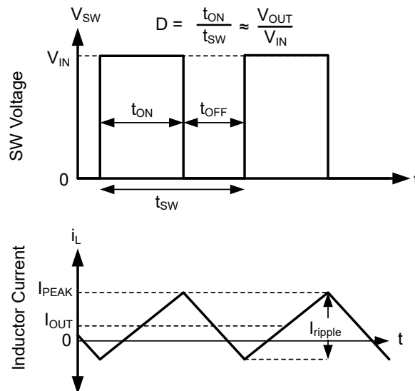
图 8-16. FPWM Mode Operation
