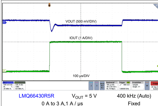
图 9-8. Load Transient
