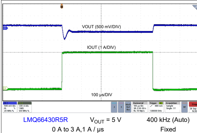
图 9-8. Load Transient
