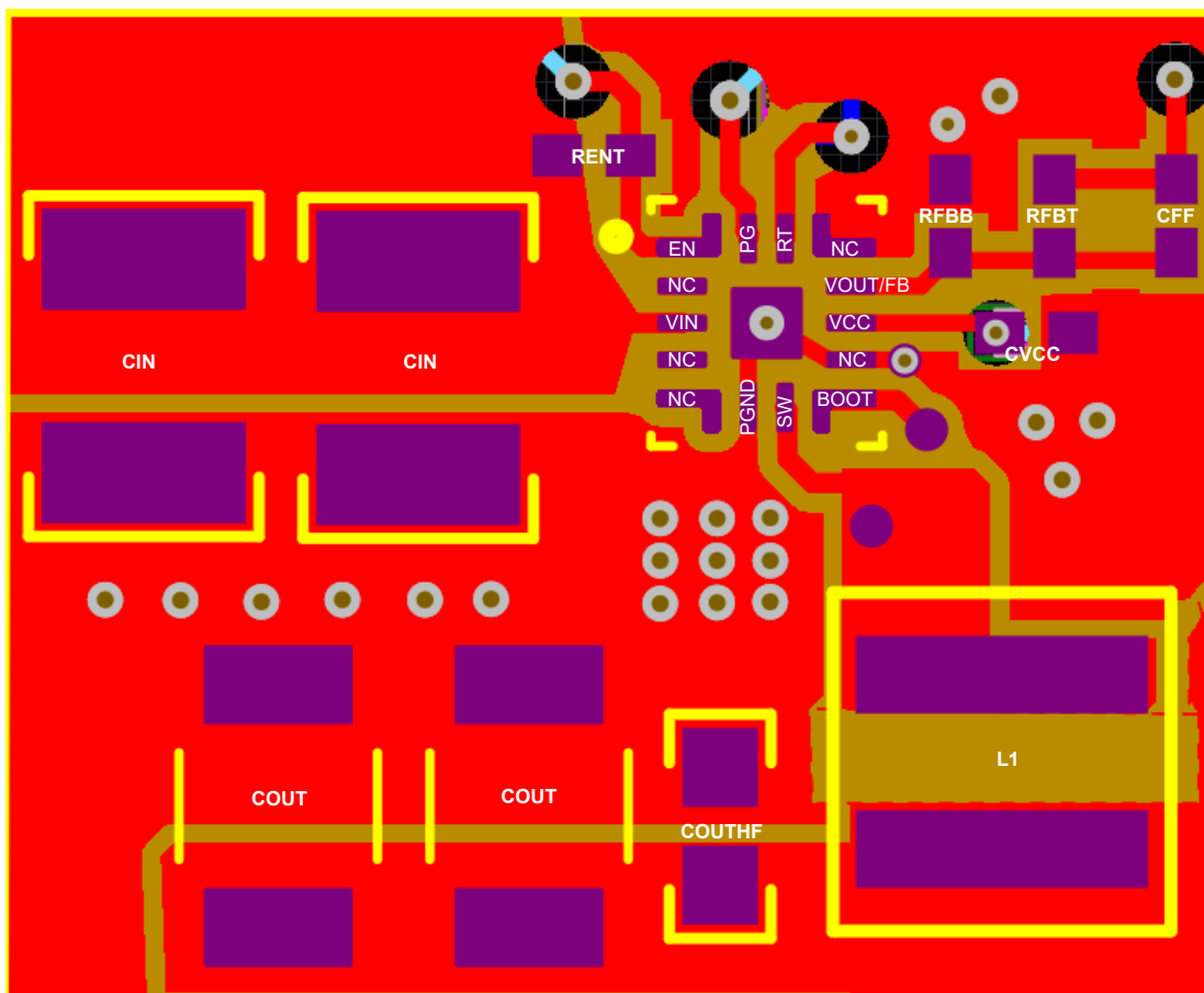
图 9-13. Example Layout
