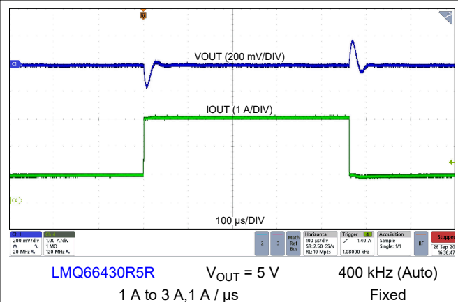
图 9-9. Load Transient
