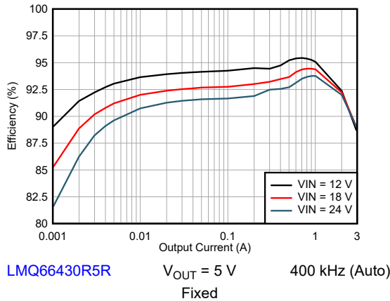
图 9-4. Efficiency
