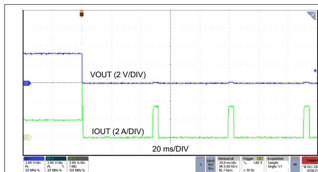
图 8-11. Hiccup Entry
