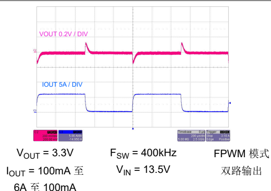
图 8-52. 负载瞬态
