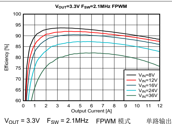
图 8-20. 效率
