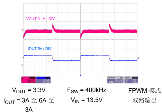
图 8-54. 负载瞬态
