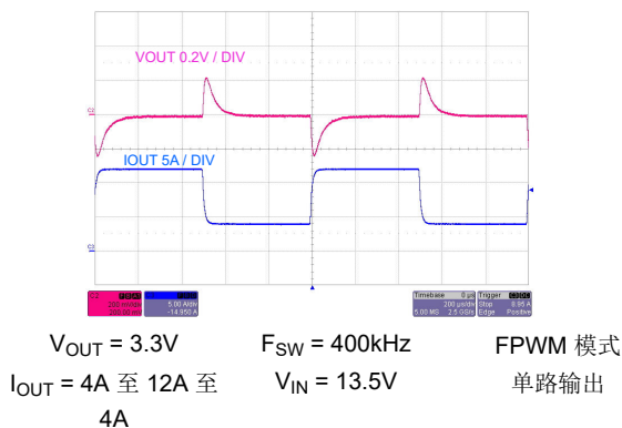
图 8-55. 负载瞬态
