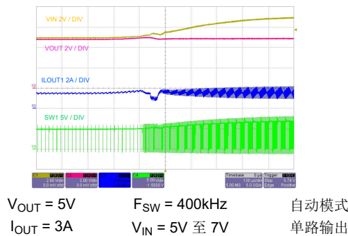
图 8-37. 压降恢复
