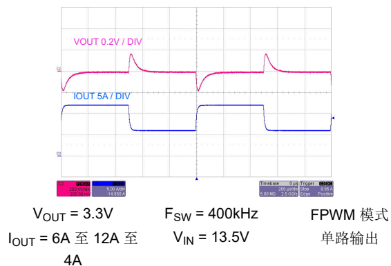
图 8-56. 负载瞬态
