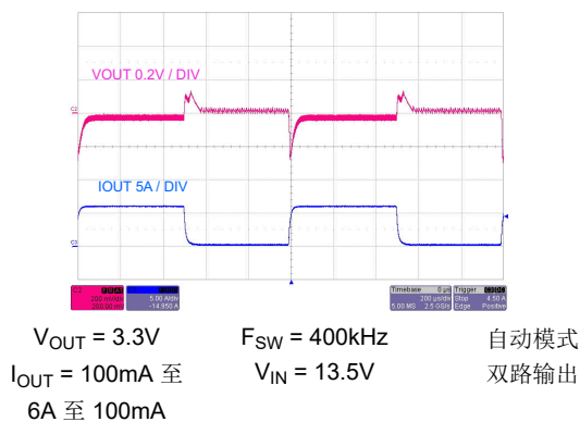
图 8-53. 负载瞬态
