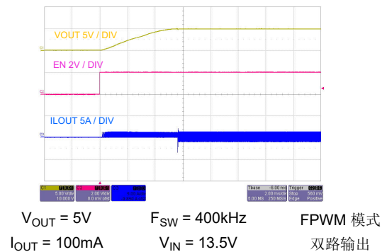
图 8-38. 在 100mA 负载下启动
