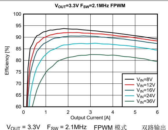
图 8-26. 效率
