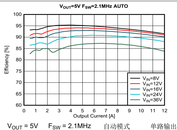
图 8-16. 效率
