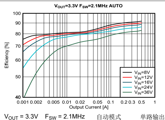
图 8-18. 效率
