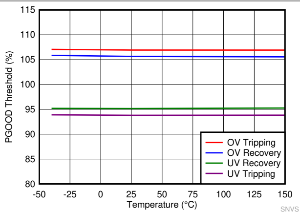
图 7-7. PGOOD 阈值
