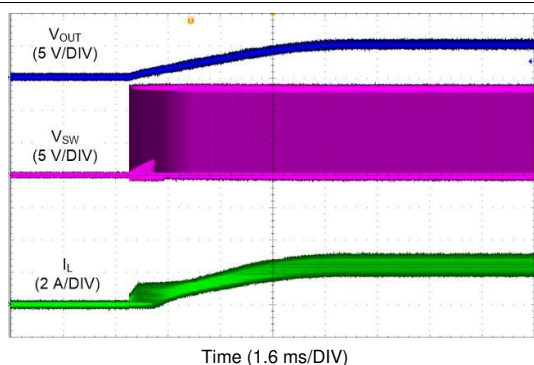
图 9-19. LMQ62440-Q1 在 3.25A 时启动
