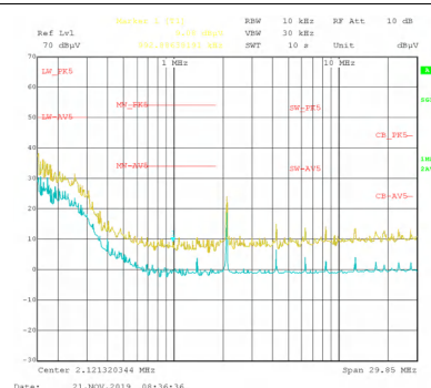
图 9-32. 辐射 EMI 对数水平与 CISPR25 限值
