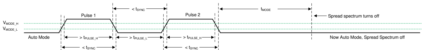
图 8-7. 在自动模式下禁用展频
