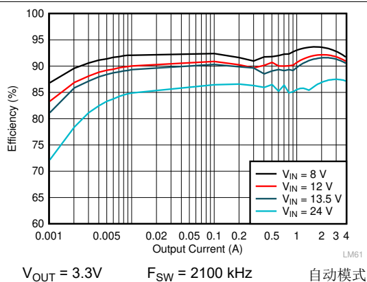
图 9-5. LMQ62440-Q1 效率
