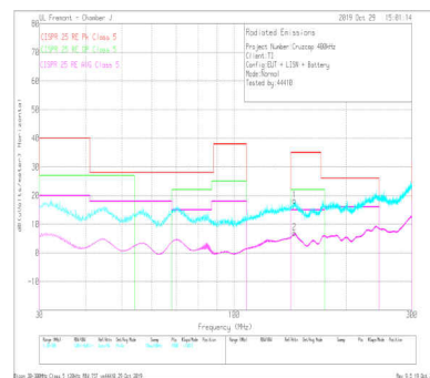
图 9-30. 辐射 EMI 双锥水平与 CISPR25 限值
