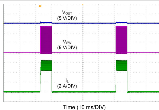
图 9-22. LMQ62440-Q1 短路性能
