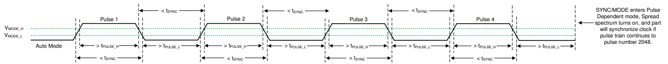
图 8-4. 从自动模式转换到脉冲相关控制
