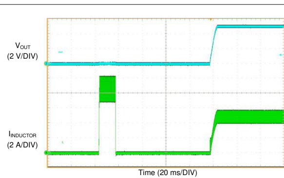
图 8-21. 短路恢复
