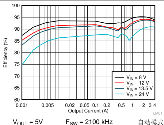
图 9-7. LMQ62440-Q1 效率
