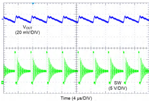
图 9-17. LMQ62440-Q1 开关波形和 V_{OUT} 纹波
