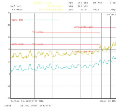
图 10-55. 传导 EMI 与 CISPR25 限值 (黄色：峰值信号，蓝色：平均信号)
