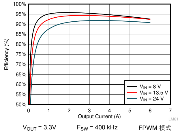
图 10-6. LMQ61460-Q1 效率
