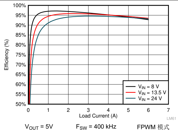
图 10-10. LMQ61460-Q1 效率
