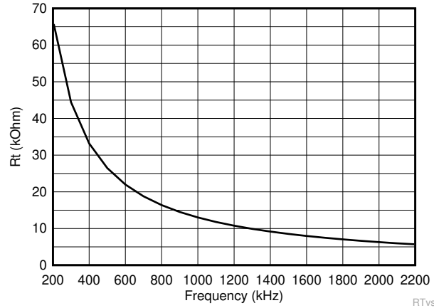
图 9-4. 设置时钟频率
