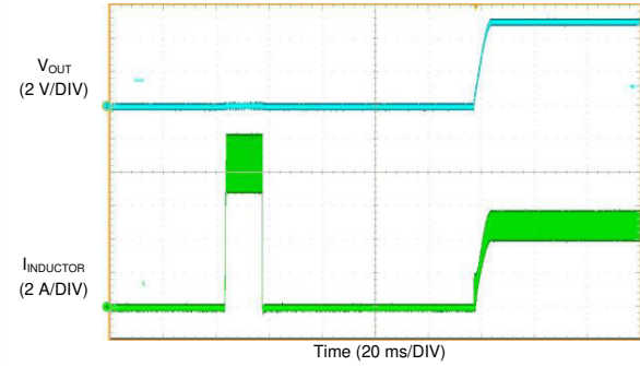
图 9-15. 短路恢复
