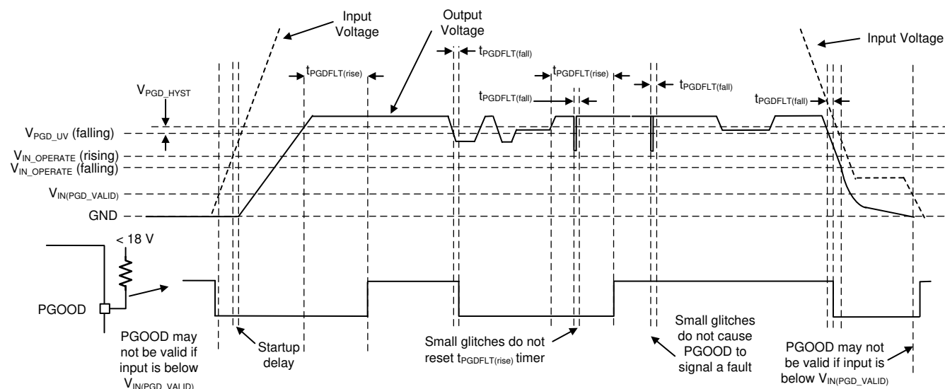
图 9-6. PGOOD 时序图 (不包括 OV 事件)
