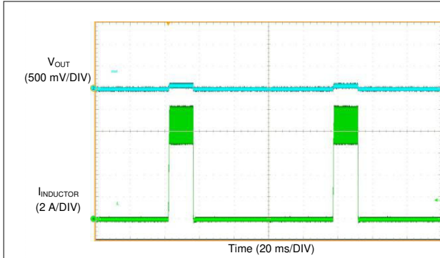
图 9-14. 断续期间的电感器电流突发
