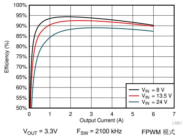
图 10-8. LMQ61460-Q1 效率
